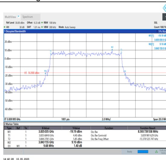
1-N77-3700-3980-PC1-30-10-M-9-CP-256QAM-Out er Full-24@0-Ant0-8.594-9.680-≤10-PASS
