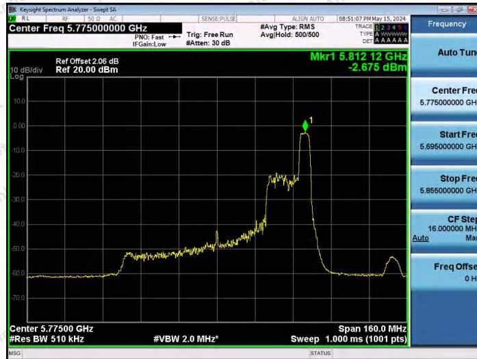
11AX80SISO-Ant1-5775-52Tone-RU52-PASS
