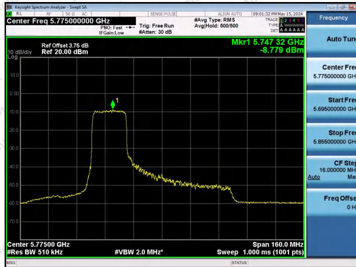
11AX80SISO-Ant1-5775-242Tone-RU61-PASS
