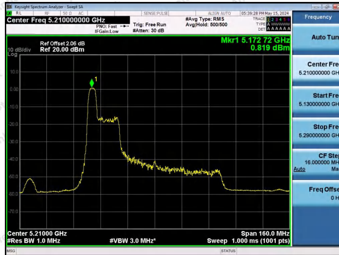
11AX80SISO-Ant1-5210-52Tone-RU37-PASS
