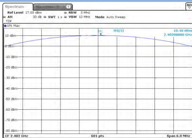
\pi/4 -DQPSK LOW CHANNEL
