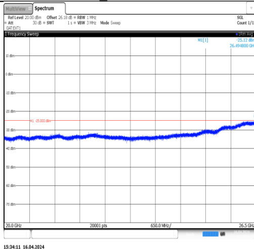
Band41_15MHz_QPSK_39725_1RB#0_20000~26500 6500 20000~26500
