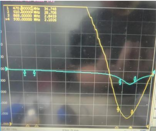
驻波图
