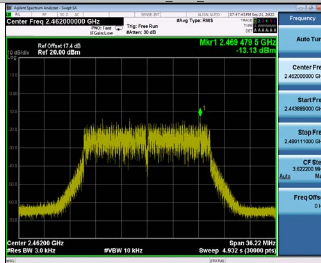
11N20SISO_Ant1_2462
