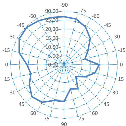
5G Ch100
