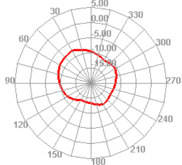
2400.000MHz H
