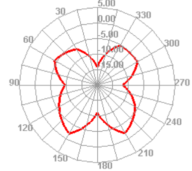
2400.000MHz E2
