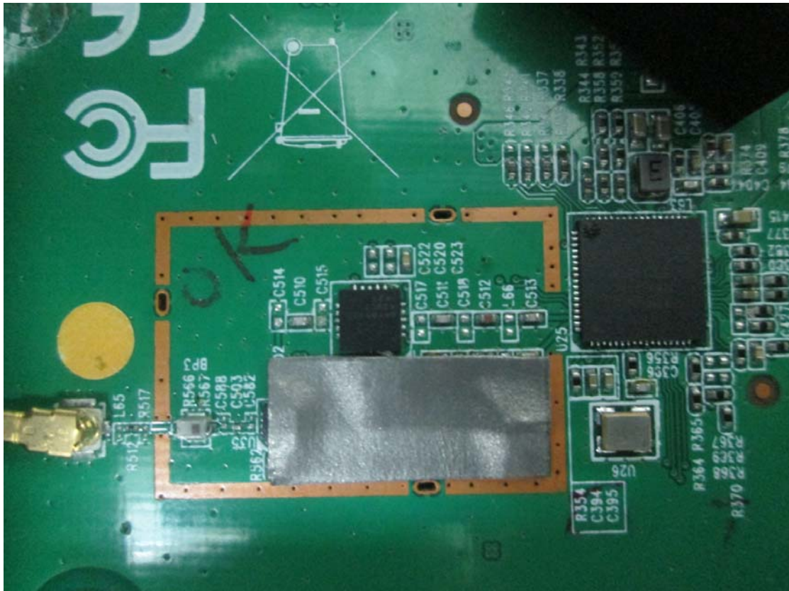
RF Module 2
