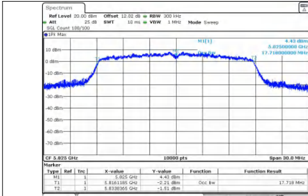
IEEE 802.11n_Channel 165_20MHz_Antenna 0
