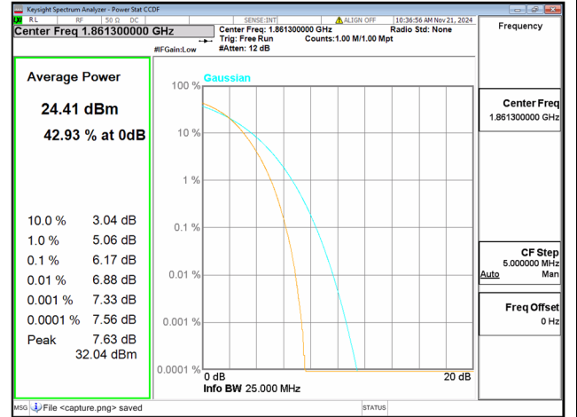
2C / 10+15MHz / Low CH / QPSK
