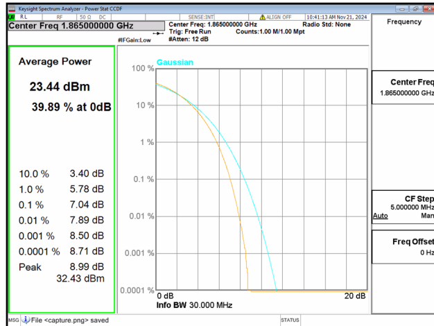
2C / 15+15MHz / Low CH / 64QAM
