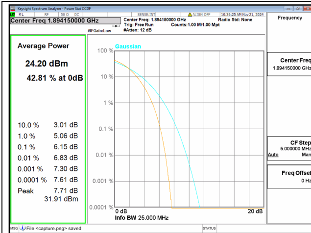
2C / 5+20MHz / High CH / QPSK
