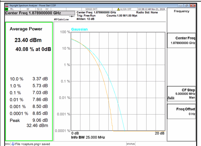
2C / 10+15MHz / Mid CH / 64QAM
