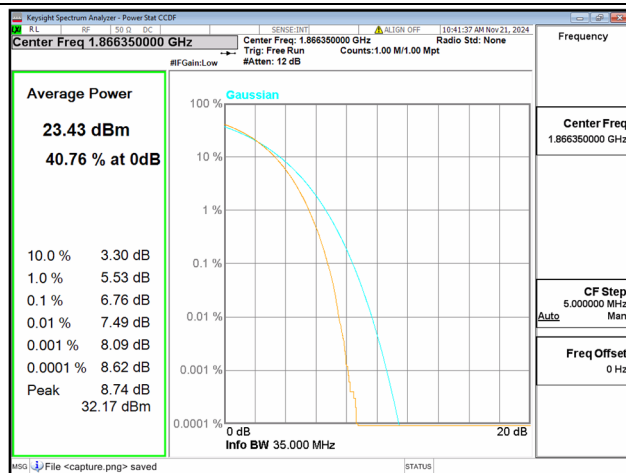
2C / 15+20MHz / Low CH / 16QAM
