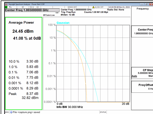
2C / 15+15MHz / Low CH / QPSK
