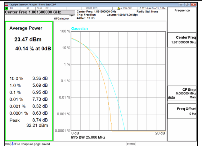
2C / 10+15MHz / Low CH / 64QAM
