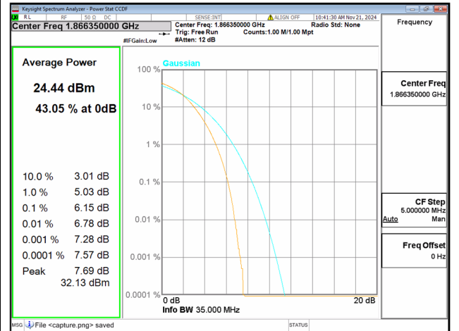
2C / 15+20MHz / Low CH / QPSK
