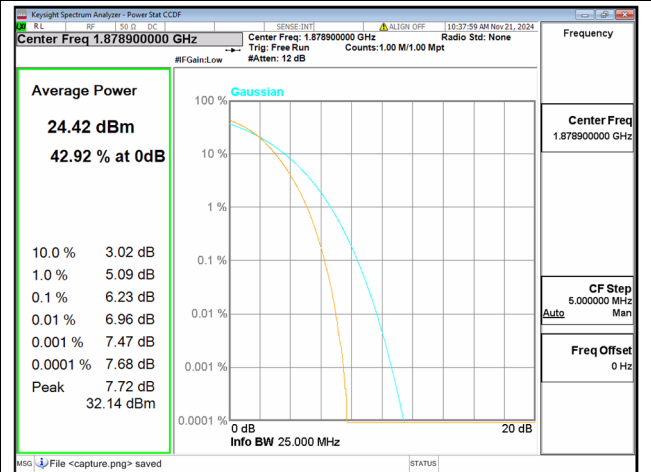
2C / 10+15MHz / Mid CH / QPSK
