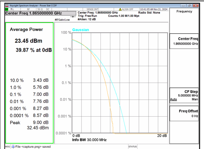
2C / 15+15MHz / Low CH / 16QAM
