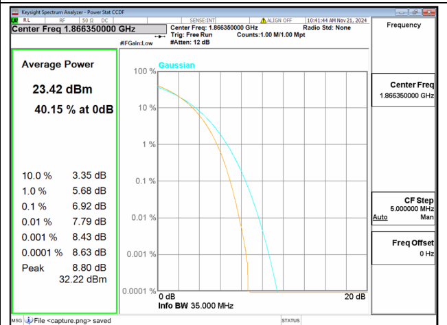
2C / 15+20MHz / Low CH / 64QAM
