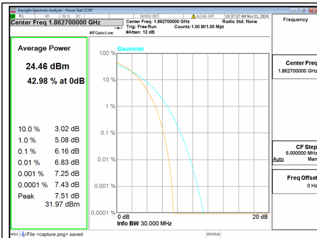
2C / 10+20MHz / Low CH / QPSK
