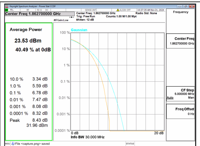
2C / 10+20MHz / Low CH / 16QAM
