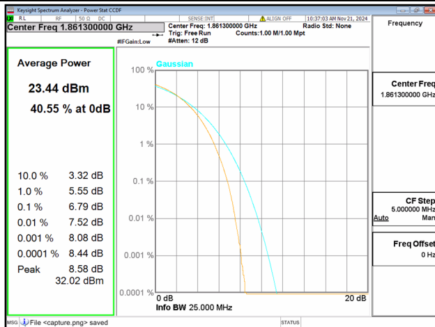
2C / 10+15MHz / Low CH / 16QAM
