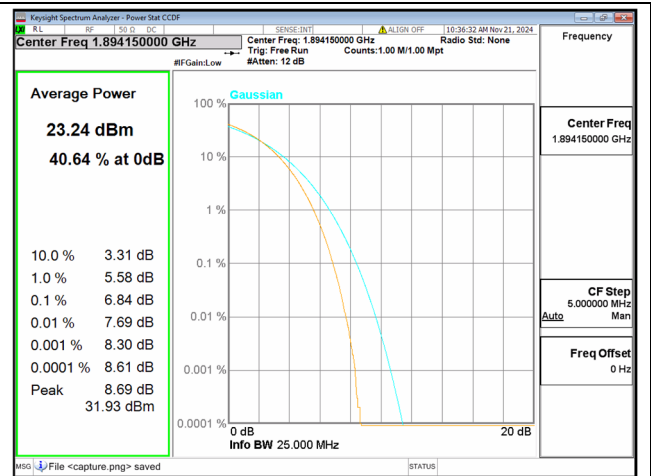
2C / 5+20MHz / High CH / 16QAM
