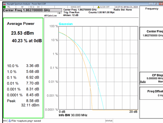
2C / 10+20MHz / Low CH / 64QAM
