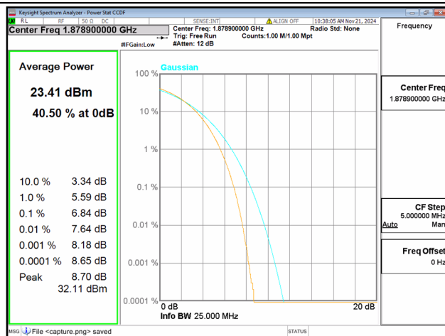
2C / 10+15MHz / Mid CH / 16QAM
