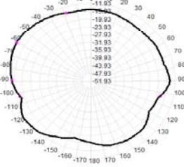
Total(H-XY), Max=-11.93dB, CrD=10.14
