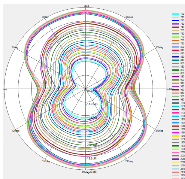
900RX/PCS1900/WCDMA B2/LTE B2 Phi=0deg
