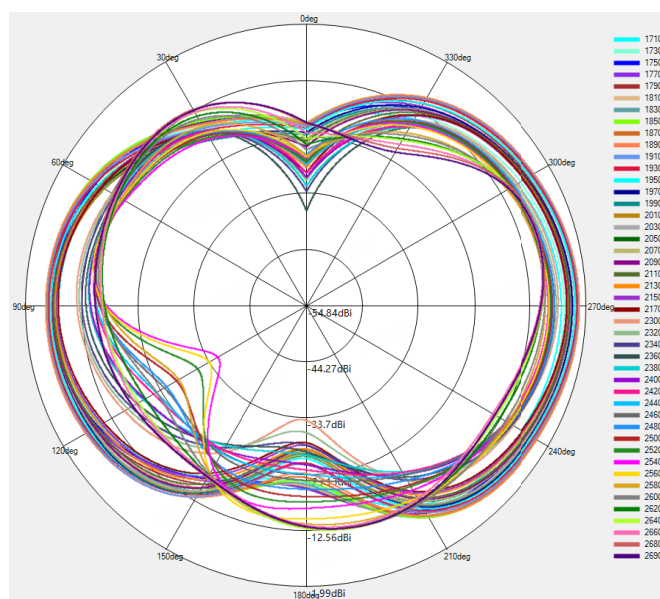
WCDMA B4/LTE B4/B7/B66 NR n7/n66 \Phi=90^\circ
