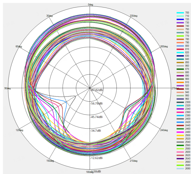
850TX/WCDMA B5/LTE B5/B20/B40 NR n5/n20/n40 Theta=90deg
