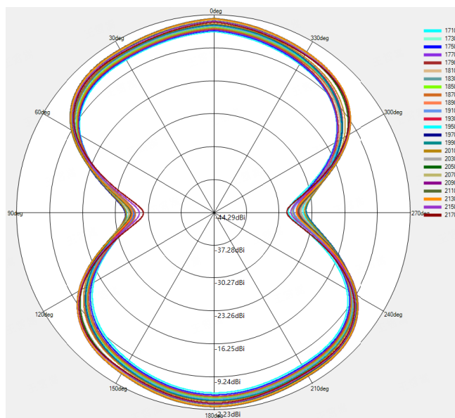
WCDMA B1/LTE B1 NR n1 \Phi=0^\circ
