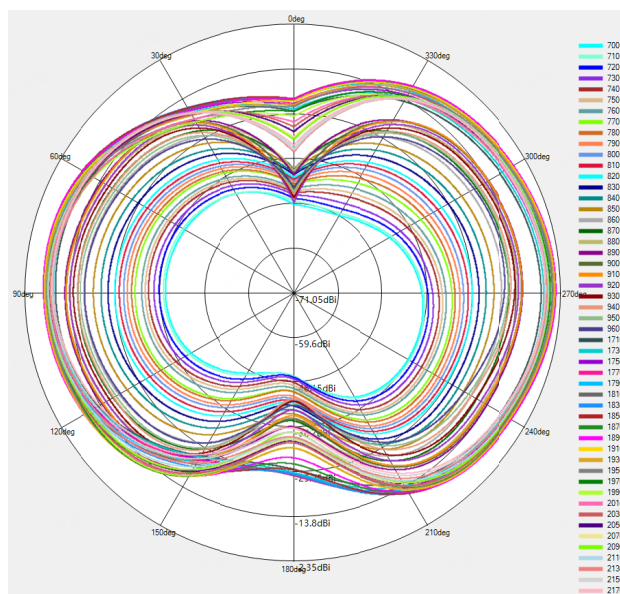
900TX/DCS1800/LTE B3 NR n3 Phi=90deg
