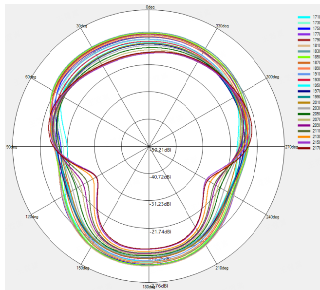
WCDMA B1/LTE B1 NR n1 Theta=90deg
