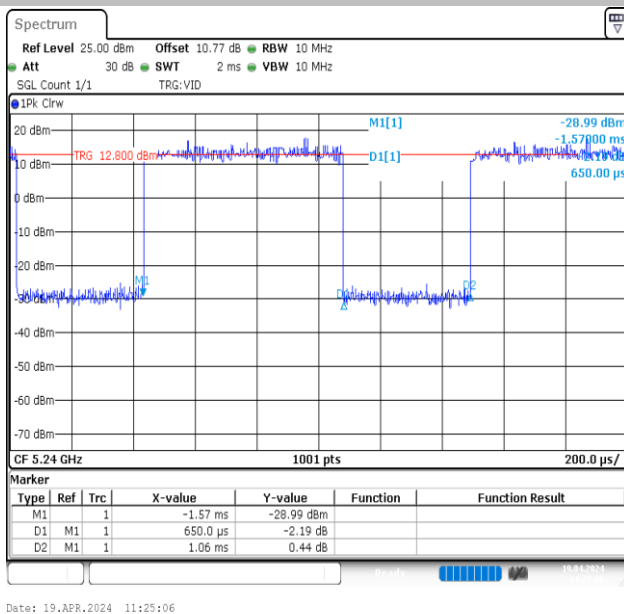
NTNV-11AX20MIMO-Ant1-5240
