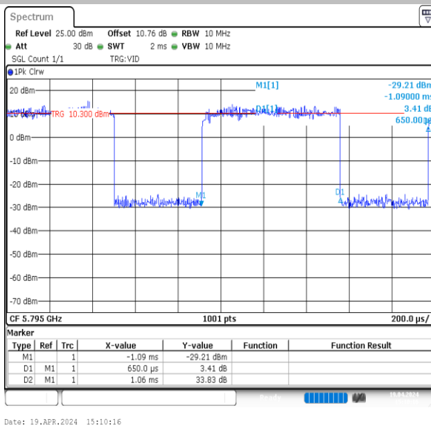
NTVN-11AX40MIMO-Ant1-5795
