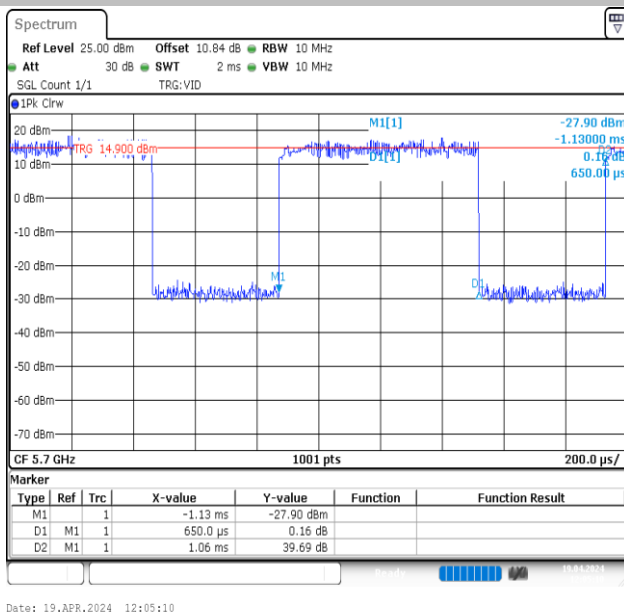
NTVN-11AX20MIMO-Ant1-5700
