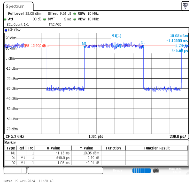
NTNV-11AX20MIMO-Ant2-5200
