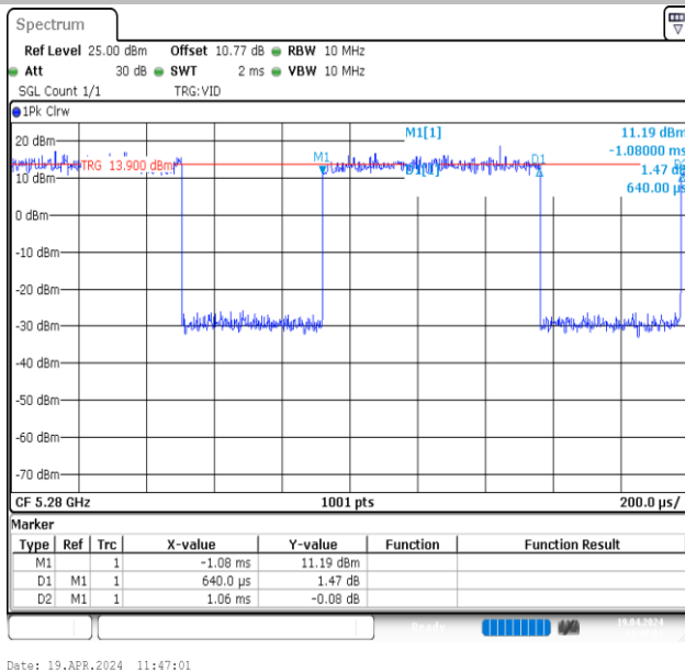
NTVN-11AX20MIMO-Ant1-5280
