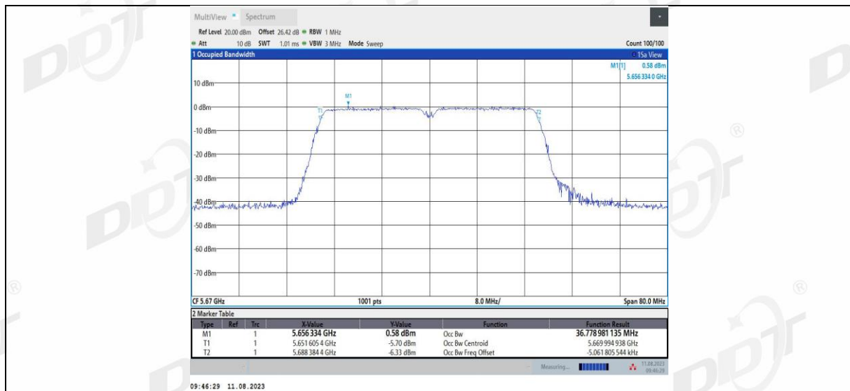
11N40MIMO_Ant2_5670
