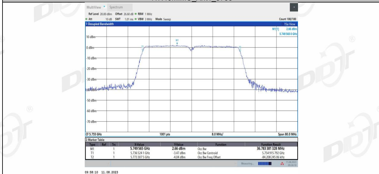
11N40MIMO_Ant2_5755
