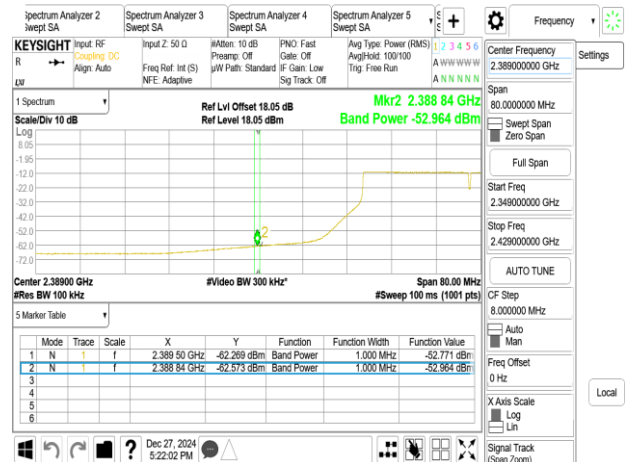
802.11be_40MHz_Chain0_2432MHz
