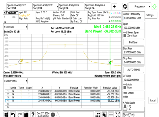
802.11be_40MHz_Chain0_2437MHz
