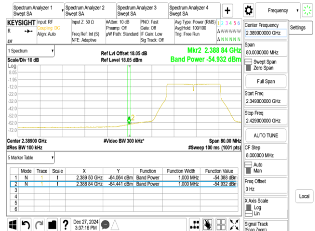
802.11be_20MHz_Chain1_2417MHz
