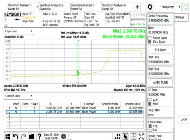
802.11be_20MHz_Chain1_2422MHz
