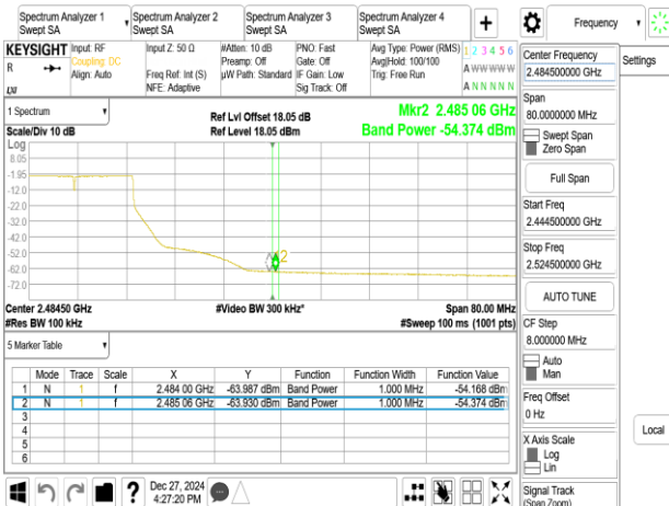
802.11be_20MHz_Chain0_2457MHz
