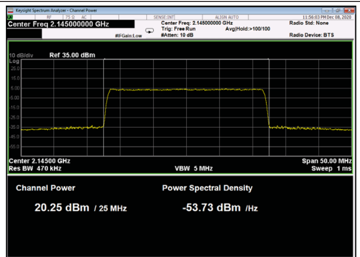
Figure 112: 64QAM 25MHz B.W.; 2145.0MHz, 30kHz
