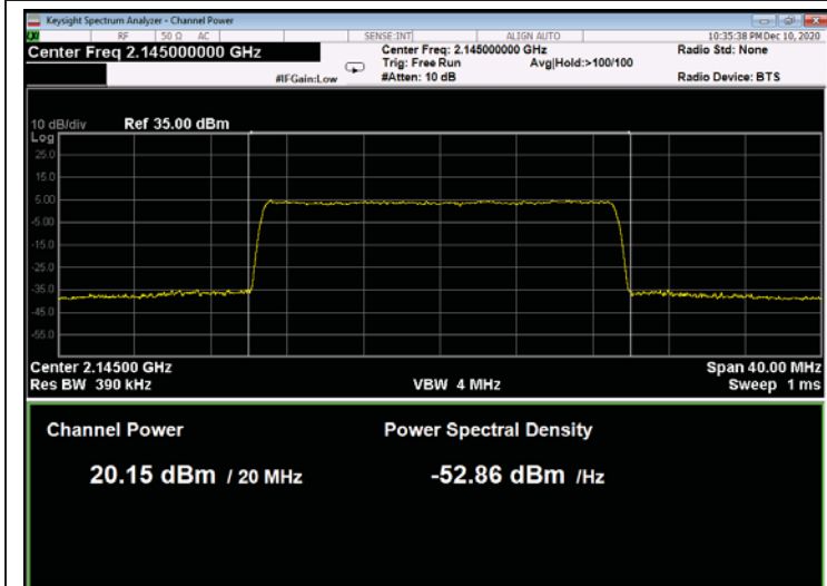
Figure 169: 256QAM 20MHz B.W.; 2145.0MHz, 30kHz
