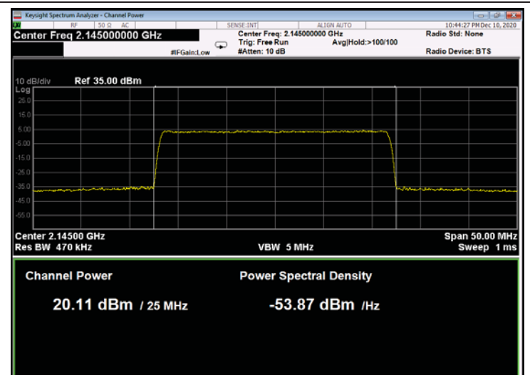
Figure 178: 256QAM 25MHz B.W.; 2145.0MHz, 30kHz
