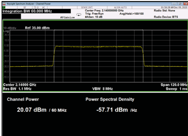
Figure 135: 64QAM 60MHz B.W.; 2140.0MHz, 30kHz
