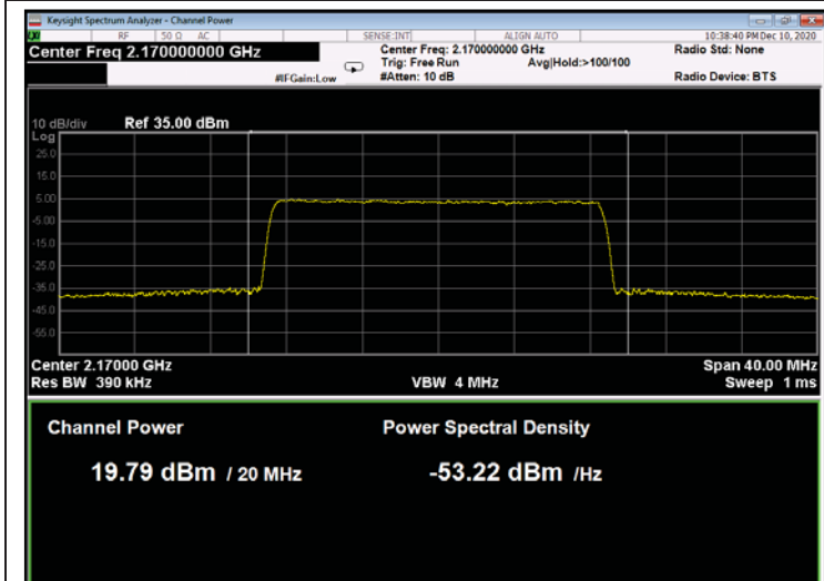
Figure 173: 256QAM 20MHz B.W.; 2170.0MHz, 60kHz
