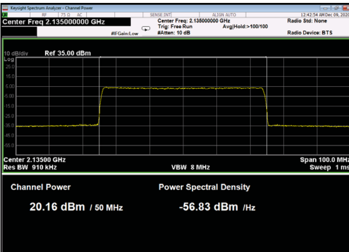
Figure 127: 64QAM 50MHz B.W.; 2135.0MHz, 30kHz
