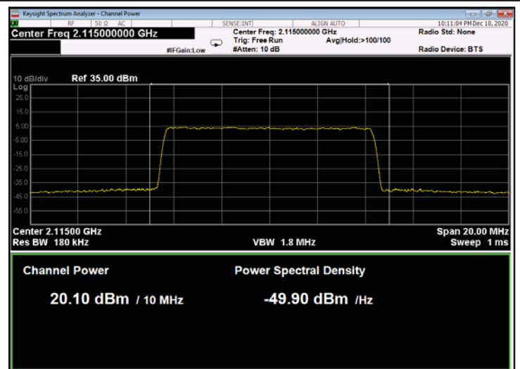
Figure 148: 256QAM 10MHz B.W.; 2115.0MHz, 30kHz
