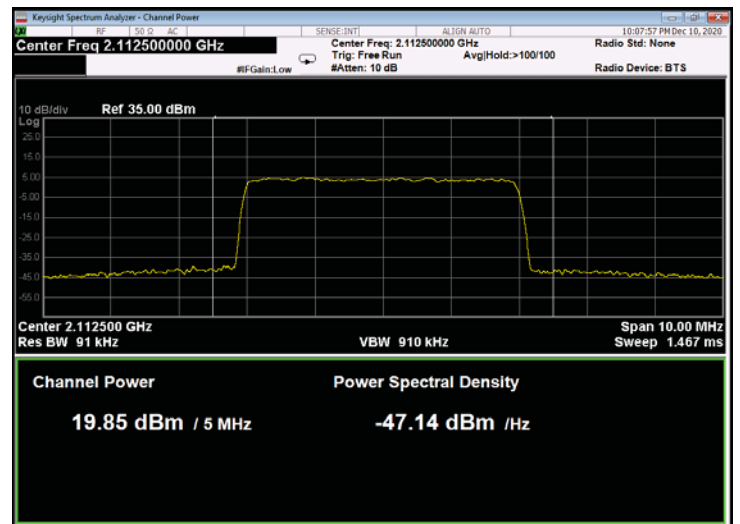
Figure 142: 256QAM 5MHz B.W.; 2112.5MHz, 30kHz
