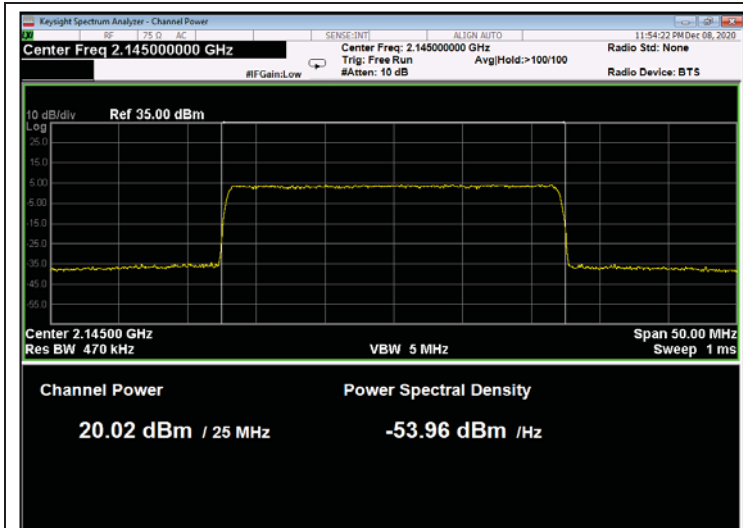
Figure 111: 64QAM 25MHz B.W.; 2145.0MHz, 15kHz
