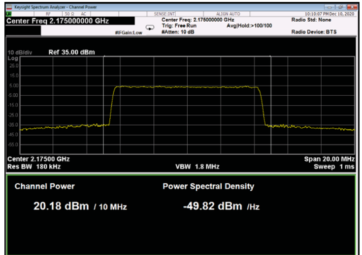
Figure 154: 256QAM 10MHz B.W.; 2175.0MHz, 30kHz
