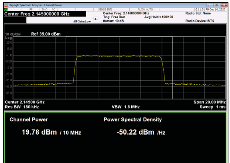
Figure 152: 256QAM 10MHz B.W.; 2145.0MHz, 60kHz
