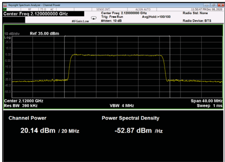
Figure 101: 64QAM 20MHz B.W.; 2120.0MHz, 60kHz
