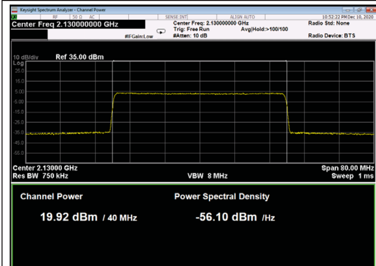
Figure 183: 256QAM 40MHz B.W.; 2130.0MHz, 15kHz
