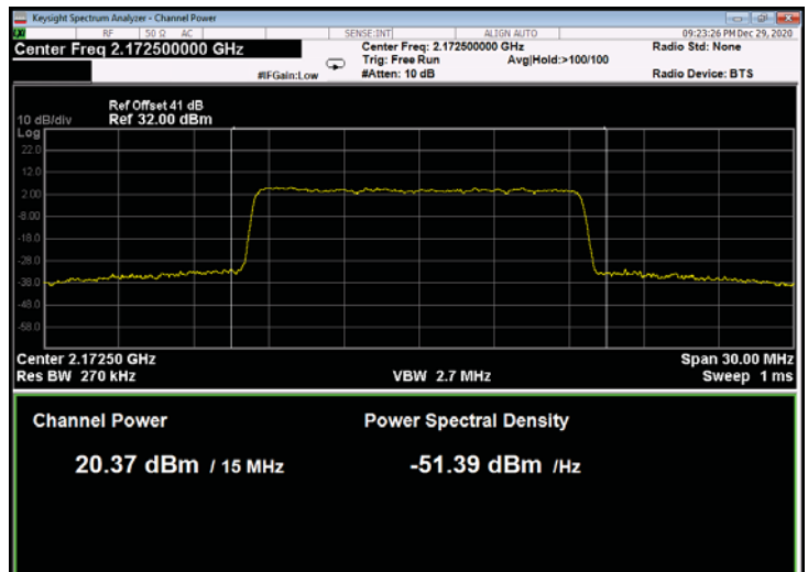
Figure 164: 256QAM 15MHz B.W.; 2172.5MHz, 60kHz
