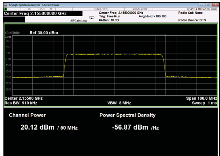
Figure 134: 64QAM 50MHz B.W.; 2155.0MHz, 60kHz
