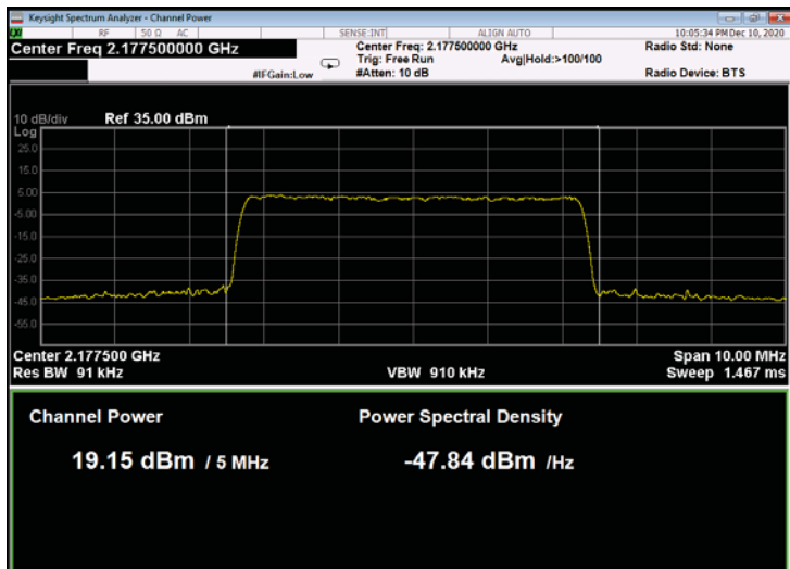
Figure 145: 256QAM 5MHz B.W.; 2177.5MHz, 15kHz
