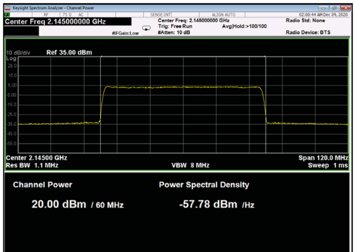
Figure 138: 64QAM 60MHz B.W.; 2145.0MHz, 60kHz
