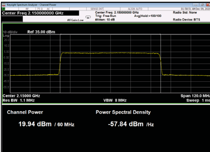
Figure 139: 64QAM 60MHz B.W.; 2150.0MHz, 30kHz
