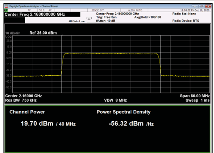
Figure 190: 256QAM 40MHz B.W.; 2160.0MHz, 30kHz
