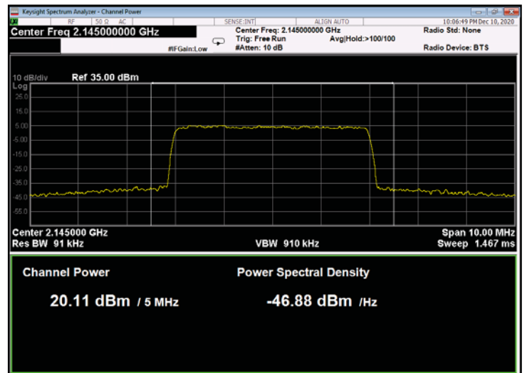
Figure 144: 256QAM 5MHz B.W.; 2145.0MHz, 30kHz
