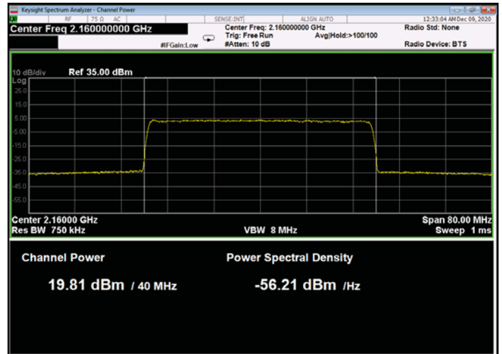
Figure 124: 64QAM 40MHz B.W.; 2160.0MHz, 30kHz
