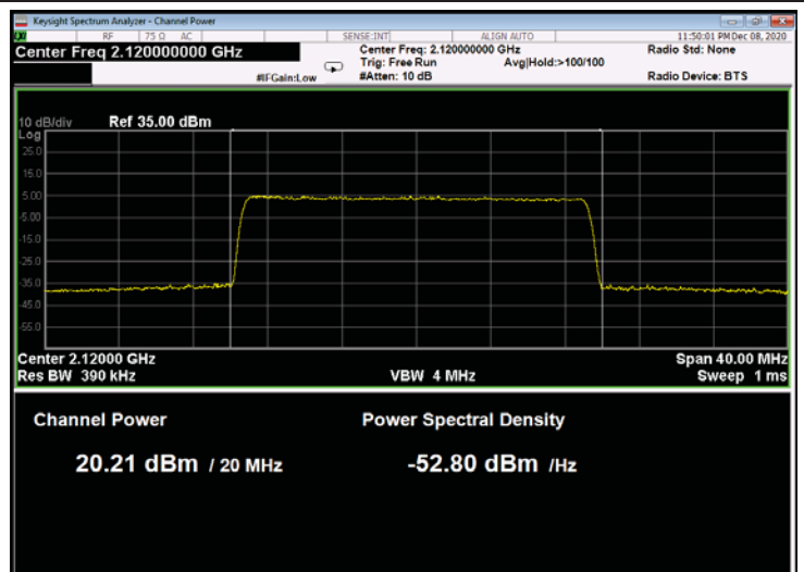
Figure 100: 64QAM 20MHz B.W.; 2120.0MHz, 30kHz
