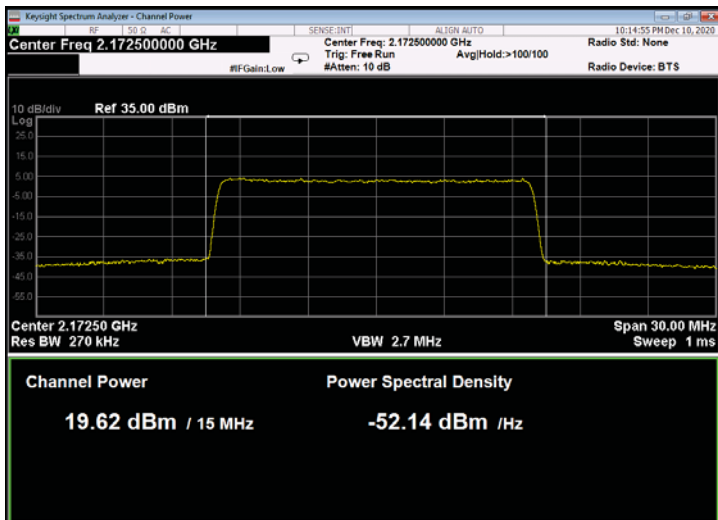
Figure 163: 256QAM 15MHz B.W.; 2172.5MHz, 30kHz
