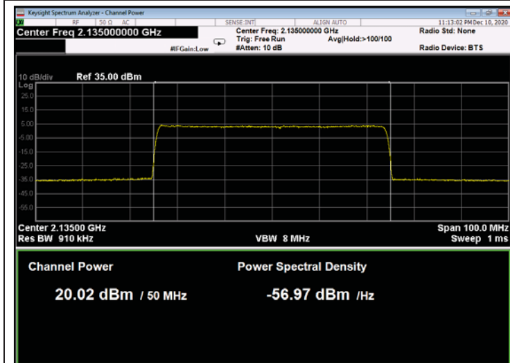
Figure 193: 256QAM 50MHz B.W.; 2135.0MHz, 30kHz
