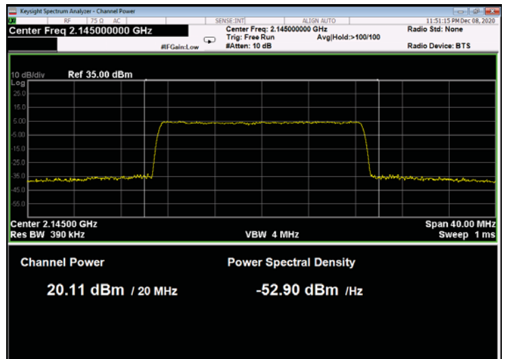
Figure 104: 64QAM 20MHz B.W.; 2145.0MHz, 60kHz
