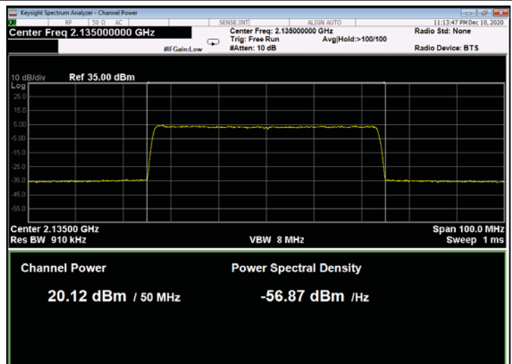
Figure 194: 64QAM 50MHz B.W.; 2135.0MHz, 60kHz
