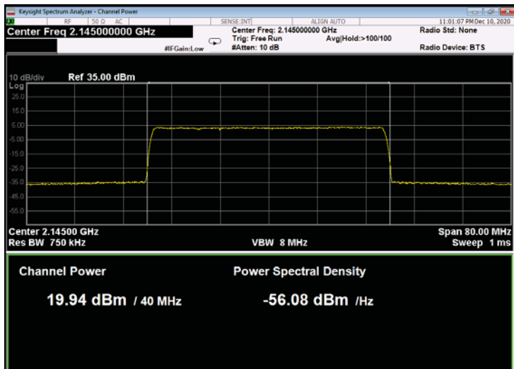
Figure 187: 256QAM 40MHz B.W.; 2145.0MHz, 30kHz
