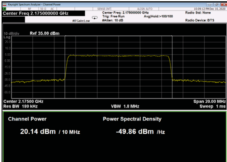
Figure 153: 256QAM 10MHz B.W.; 2175.0MHz, 15kHz
