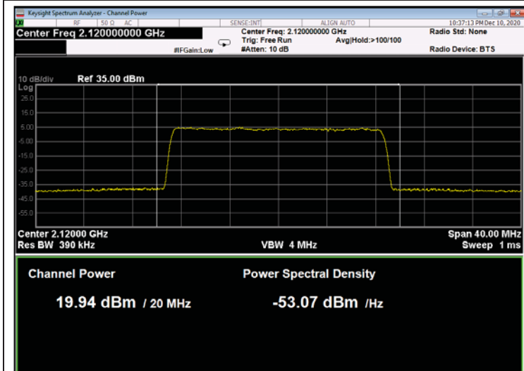
Figure 167: 256QAM 20MHz B.W.; 2120.0MHz, 60kHz
