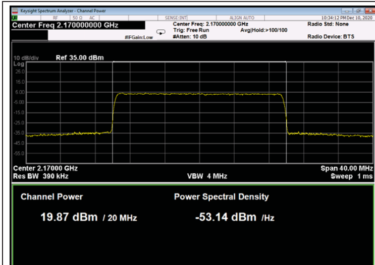
Figure 171: 256QAM 20MHz B.W.; 2170.0MHz, 15kHz
