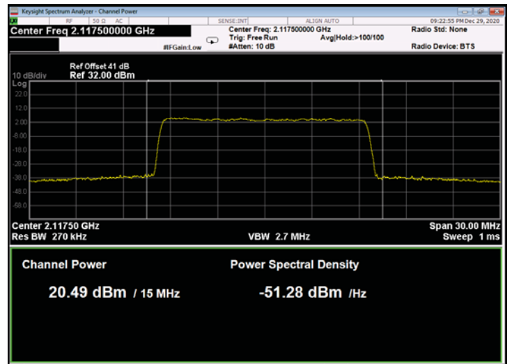
Figure 158: 256QAM 15MHz B.W.; 2117.5MHz, 60kHz
