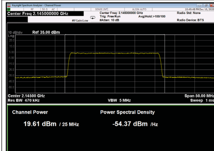
Figure 179: 256QAM 25MHz B.W.; 2145.0MHz, 60kHz
