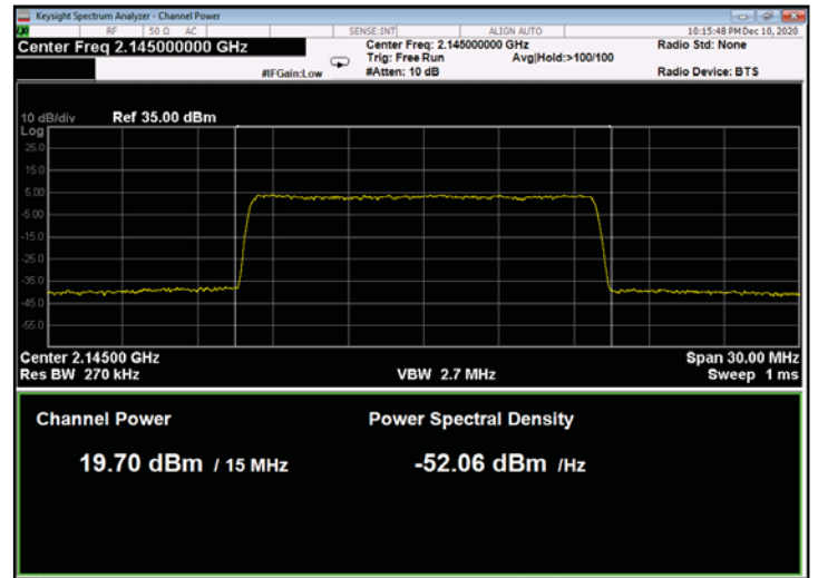
Figure 160: 256QAM 15MHz B.W.; 2145.0MHz, 30kHz
