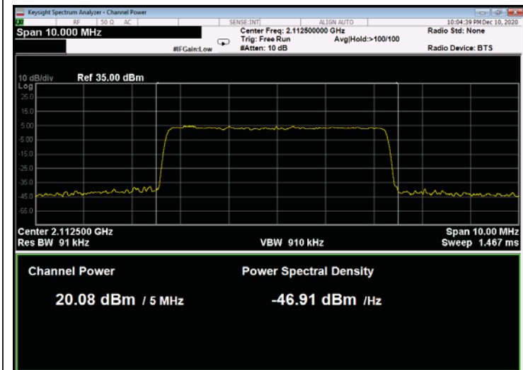
Figure 141: 256QAM 5MHz B.W.; 2112.5MHz, 15kHz
