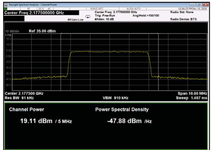
Figure 146: 256QAM 5MHz C.S.; 2177.5MHz, 30kHz
