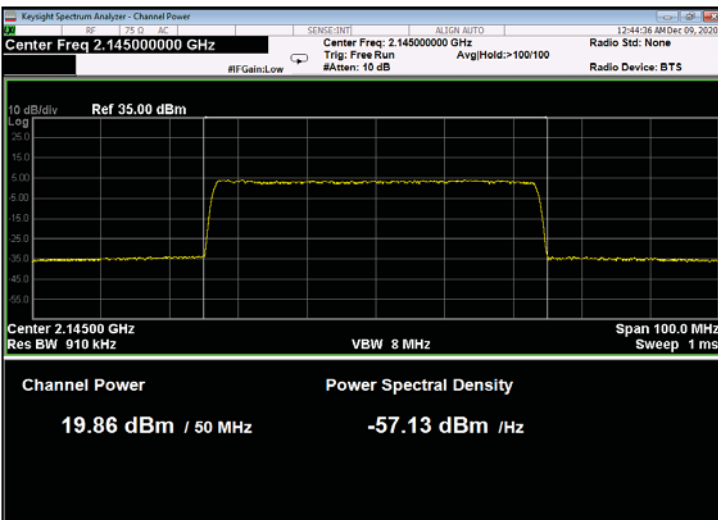
Figure 131: 64QAM 50MHz B.W.; 2145.0MHz, 60kHz
