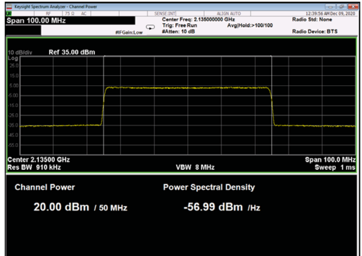
Figure 126: 64QAM 50MHz B.W.; 2135.0MHz, 15kHz
