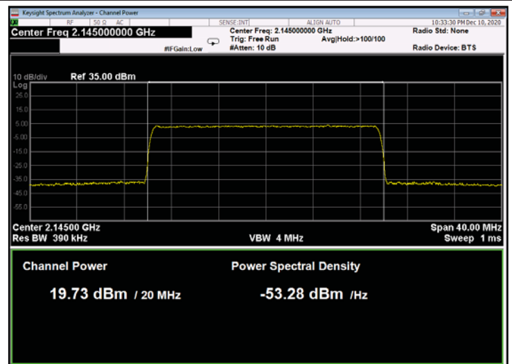
Figure 168: 256QAM 20MHz B.W.; 2145.0MHz, 15kHz
