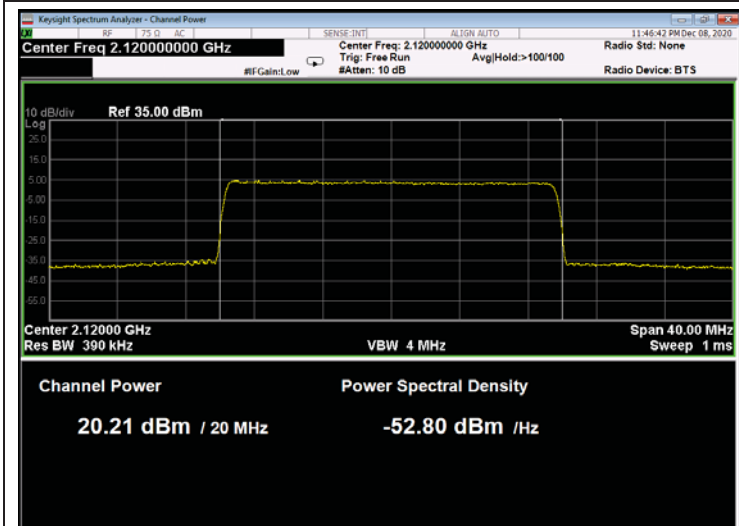
Figure 99: 64QAM 20MHz B.W.; 2120.0MHz, 15kHz
