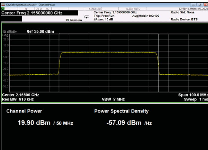
Figure 133: 64QAM 50MHz B.W.; 2155.0MHz, 30kHz
