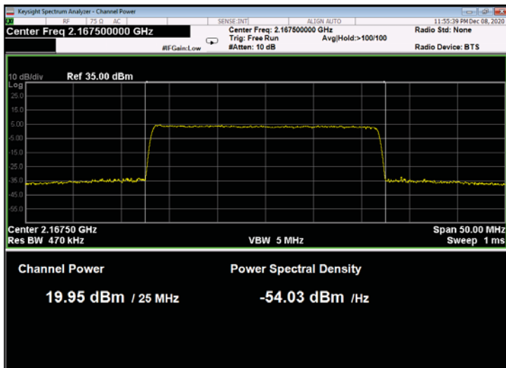
Figure 115: 64QAM 25MHz B.W.; 2167.5MHz, 30kHz
