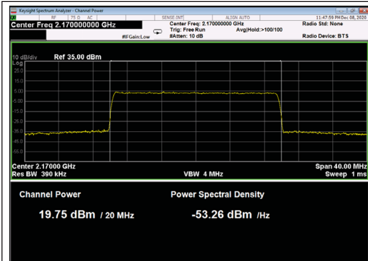
Figure 105: 64QAM 20MHz B.W.; 2170.0MHz, 15kHz
