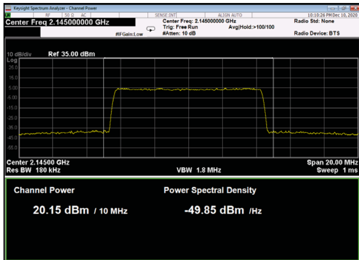
Figure 151: 256QAM 10MHz B.W.; 2145.0MHz, 30kHz
