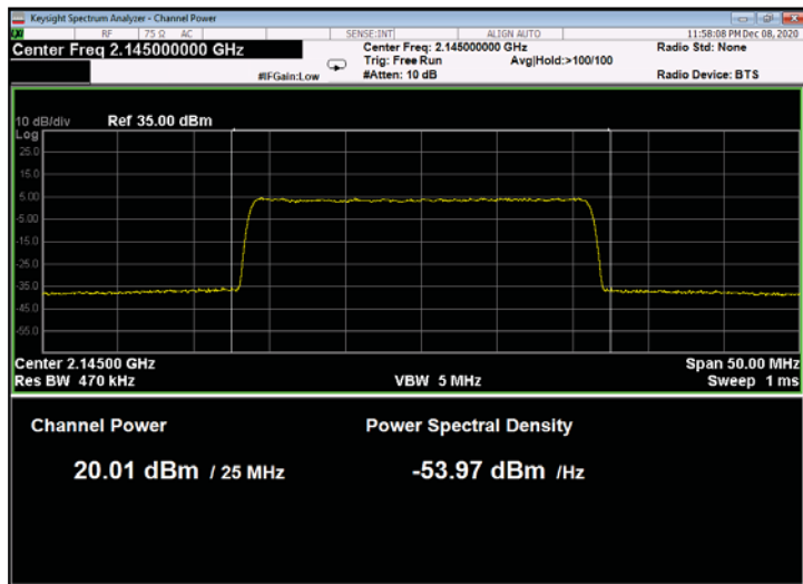
Figure 113: 64QAM 25MHz B.W.; 2145.0MHz, 60kHz
