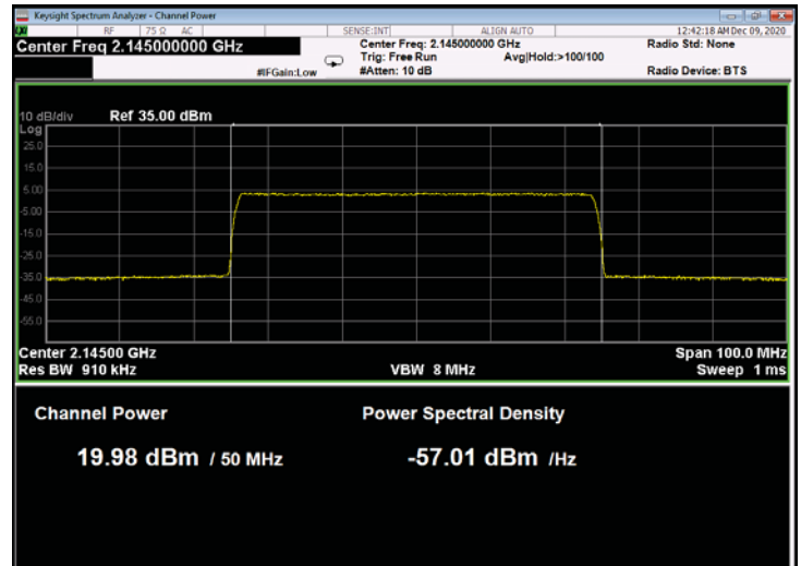
Figure 130: 64QAM 50MHz B.W.; 2145.0MHz, 30kHz
