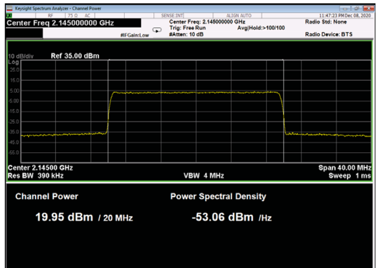
Figure 102: 64QAM 20MHz B.W.; 2145.0MHz, 15kHz
