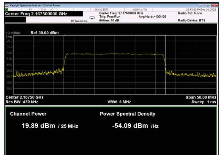
Figure 180: 256QAM 25MHz B.W.; 2167.5MHz, 15kHz
