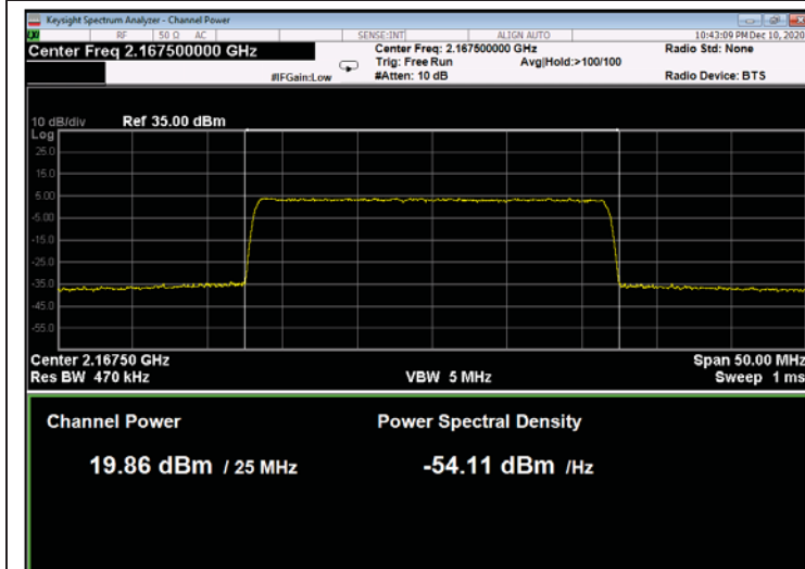
Figure 181: 256QAM 25MHz B.W.; 2167.5MHz, 30kHz
