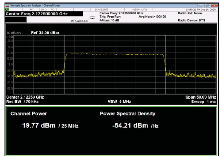
Figure 174: 256QAM 25MHz B.W.; 2122.5MHz, 15kHz
