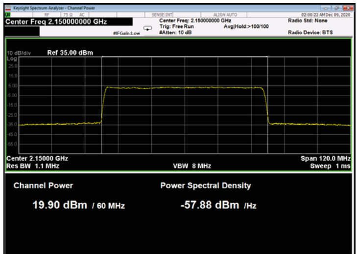
Figure 140: 64QAM 60MHz B.W.; 2150.0MHz, 60kHz
