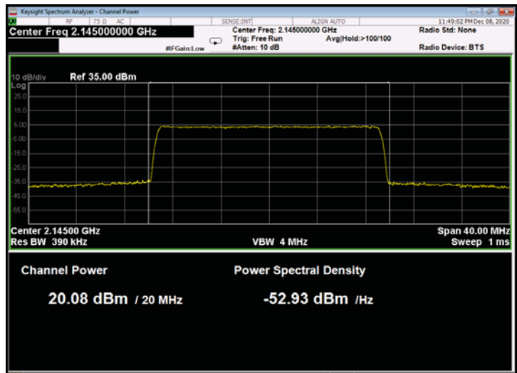
Figure 103: 64QAM 20MHz B.W.; 2145.0MHz, 30kHz
