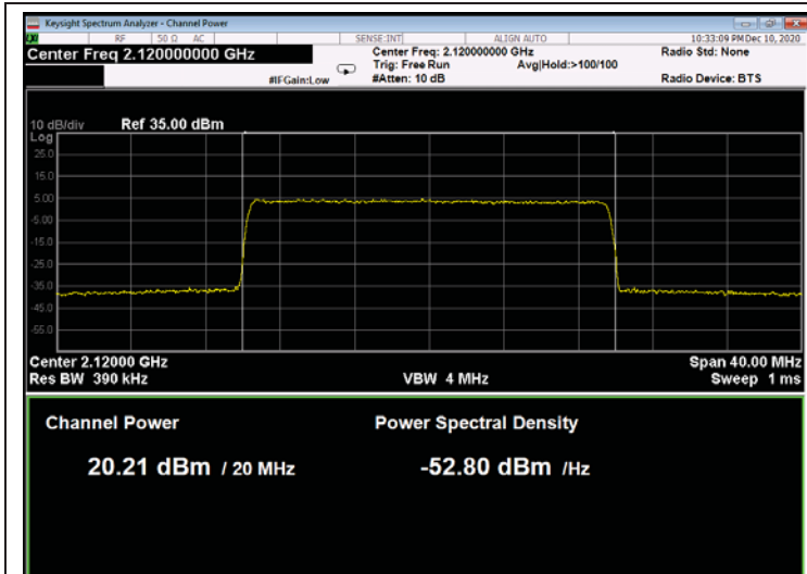
Figure 165: 256QAM 20MHz B.W.; 2120.0MHz, 15kHz
