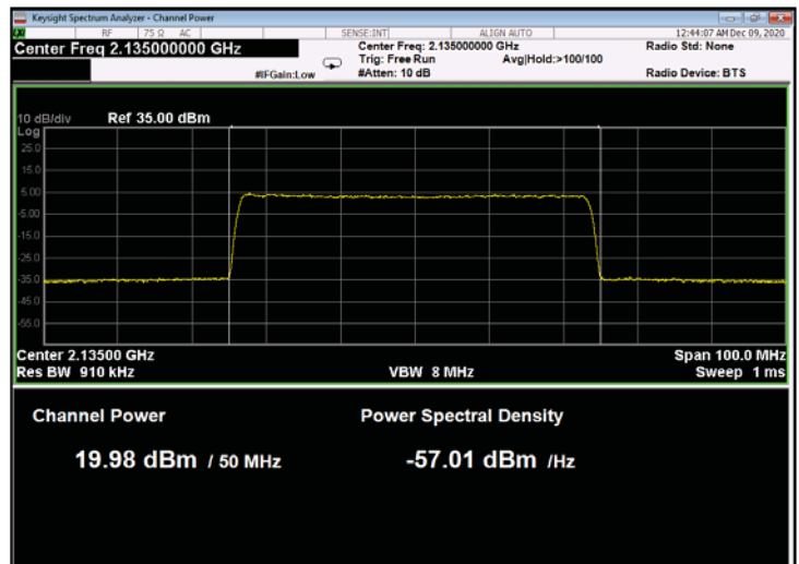
Figure 128: 64QAM 50MHz B.W.; 2135.0MHz, 60kHz
