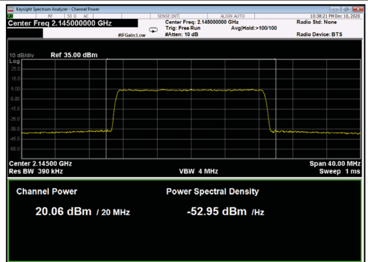
Figure 170: 256QAM 20MHz B.W.; 2145.0MHz, 60kHz
