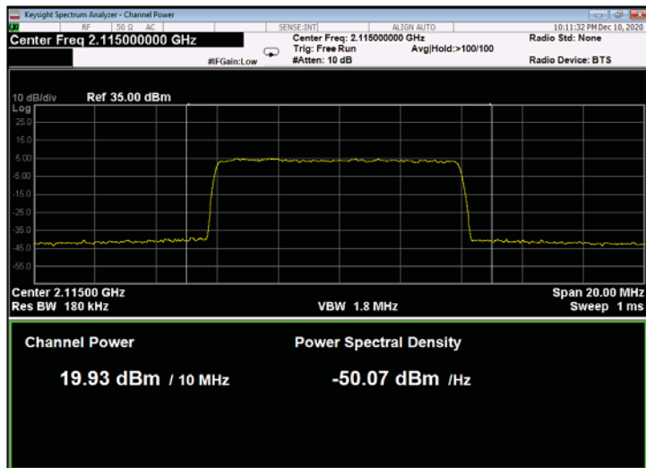
Figure 149: 256QAM 10MHz B.W.; 2115.0MHz, 60kHz
