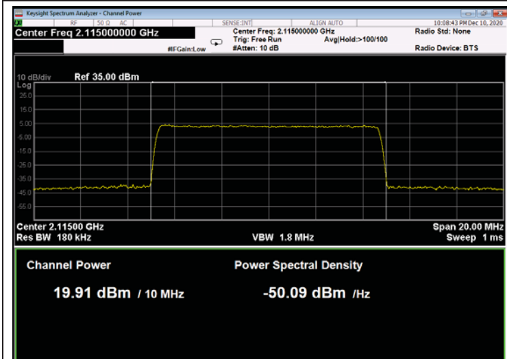
Figure 147: 256QAM 10MHz B.W.; 2115.0MHz, 15kHz
