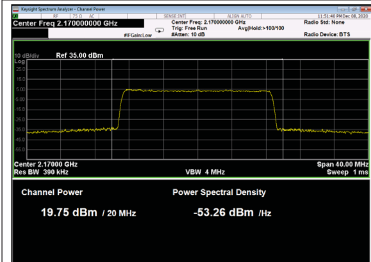
Figure 107: 64QAM 20MHz B.W.; 2170.0MHz, 60kHz
