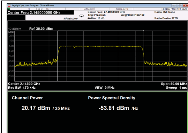
Figure 177: 256QAM 25MHz B.W.; 2145.0MHz, 15kHz
