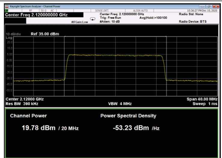
Figure 166: 256QAM 20MHz B.W.; 2120.0MHz, 30kHz
