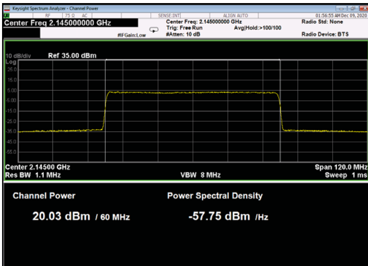
Figure 137: 64QAM 60MHz B.W.; 2145.0MHz, 30kHz
