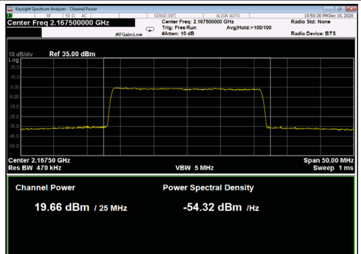
Figure 182: 256QAM 25MHz B.W.; 2167.5MHz, 60kHz
