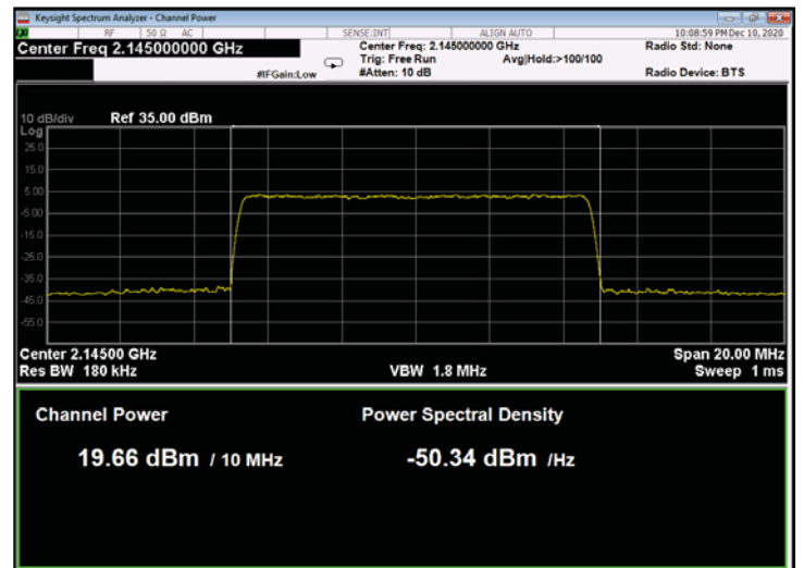
Figure 150: 256QAM 10MHz B.W.; 2145.0MHz, 15kHz
