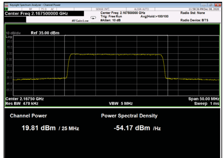
Figure 116: 64QAM 25MHz B.W.; 2167.5MHz, 60kHz
