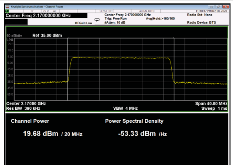
Figure 106: 64QAM 20MHz B.W.; 2170.0MHz, 30kHz
