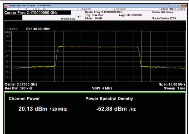
Figure 172: 256QAM 20MHz B.W.; 2170.0MHz, 30kHz
