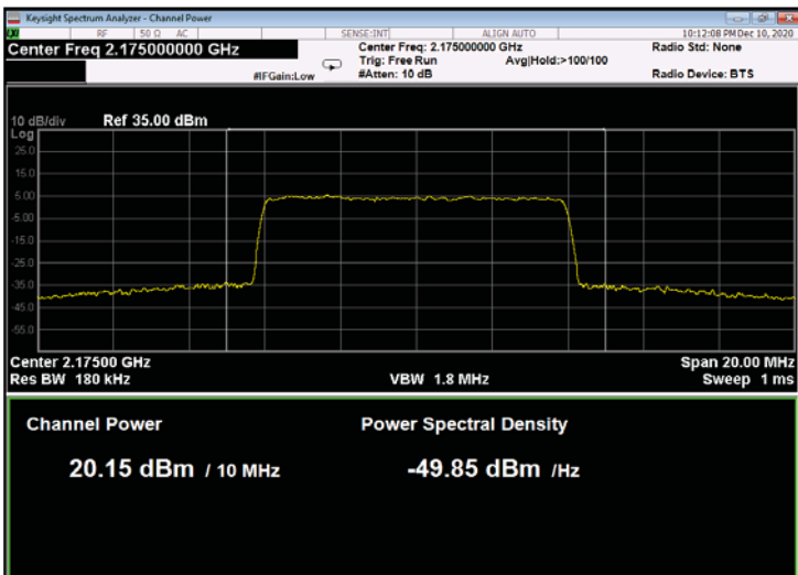
Figure 155: 256QAM 10MHz B.W.; 2175.0MHz, 60kHz
