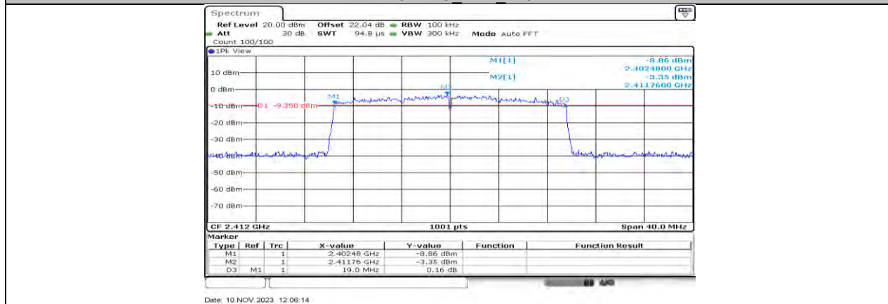
11AX20MIMO_Ant1_2412
