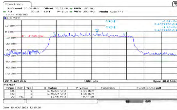
11AX20MIMO_Ant2_2462
