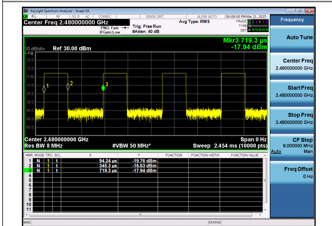
BLE_2M-Ant1-2480
