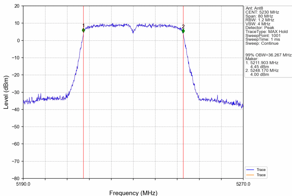
802.11n(HT40)_HCH_5230MHz_Ant8_NTNV
