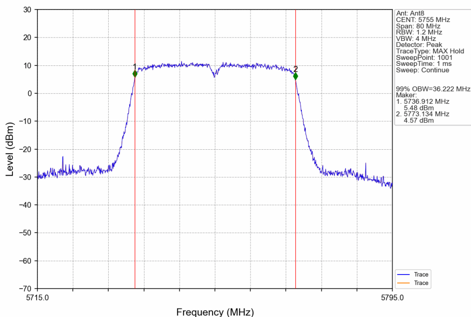
802.11n(HT40)_LCH_5755MHz_Ant8_NTNV
