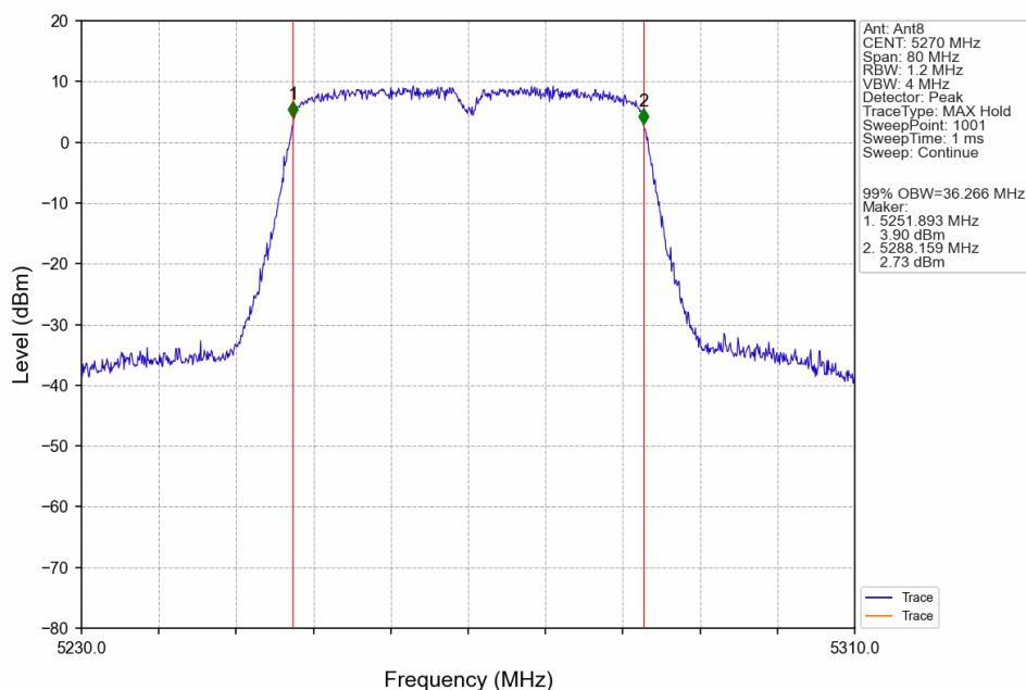
802.11ac(VHT40)_LCH_5270MHz_Ant8_NTNV
