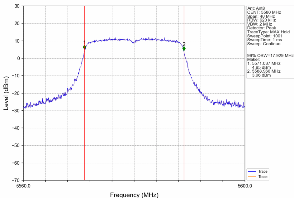
802.11n(HT20)_MCH_5580MHz_Ant8_NTNV
