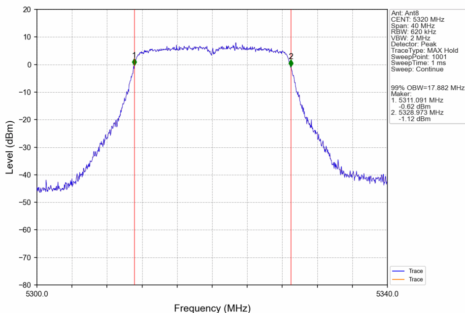
802.11n(HT20)_HCH_5320MHz_Ant8_NTNV
