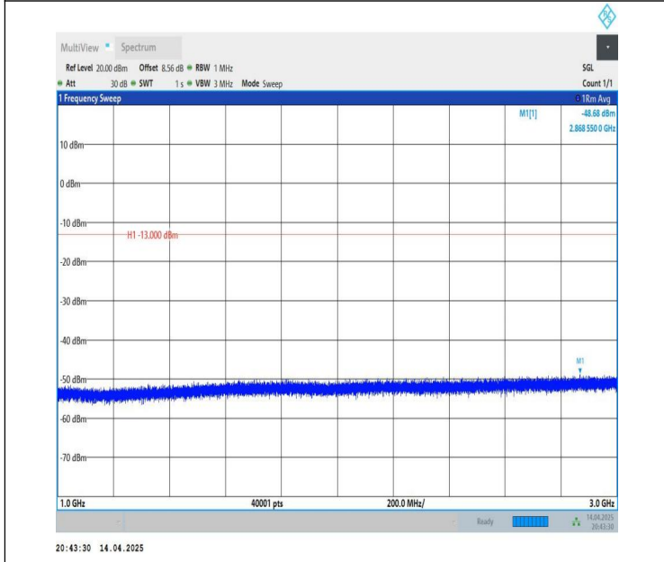
Band26(824-849)-10MHz-QPSK-26990-1RB#49-1000~3000-PAS
