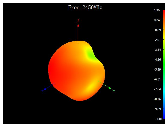
2500MHz 3D
