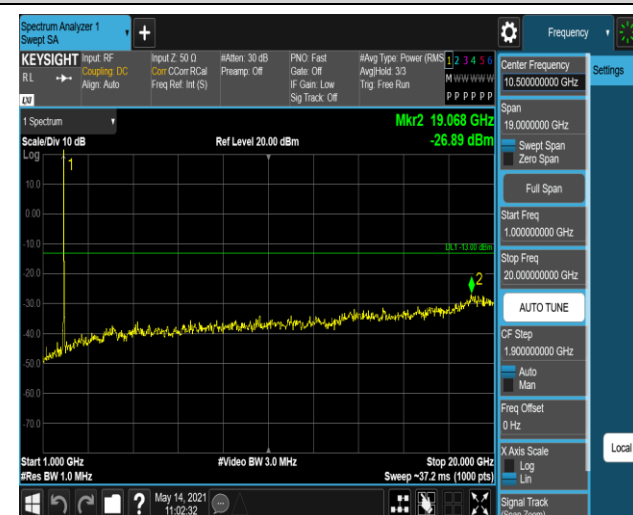
Band2-20MHz-QPSK-18900-1RB#0-Range2:1000~200
