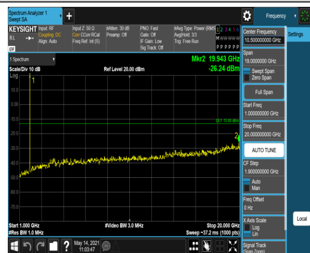
Band2-20MHz-16QAM-19100-1RB#0-Range2:1000~20
