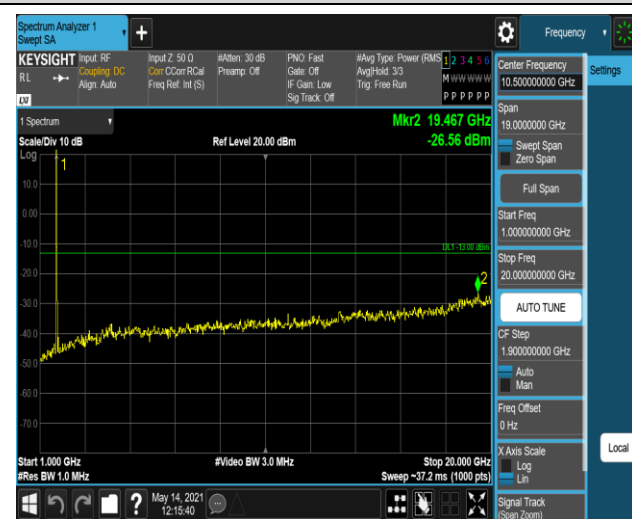
Band4-20MHz-QPSK-20175-1RB#0-Range2:1000~200
