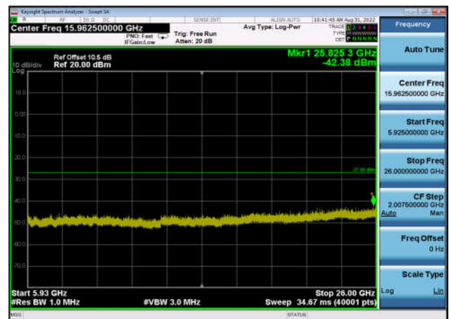
U-NII-3 ,Plot 3,5925MHz~26000MHz-802. 11ax(20MHz),5825MHz,Ant1
