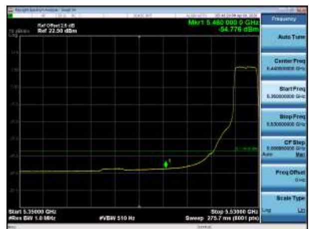
5520MHz AV
