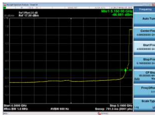
5180MHz AV
