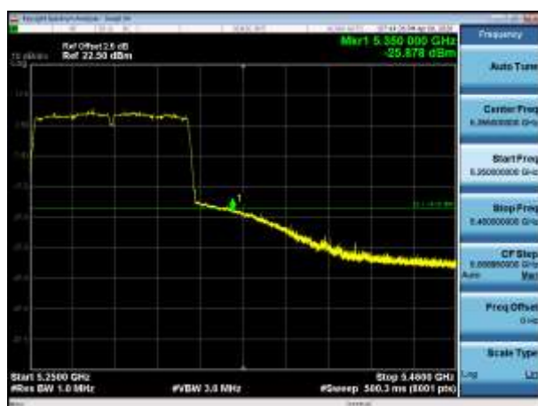
5290MHz PK
