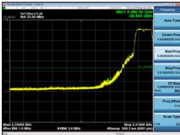
5500MHz PK
