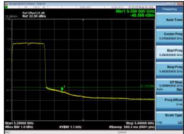
5310MHz AV
