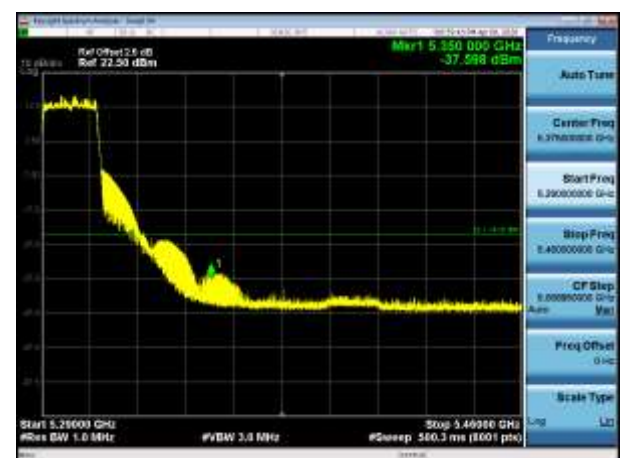
5300MHz PK
