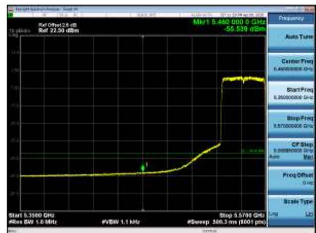
5550MHz AV
