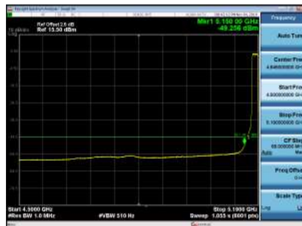
5180MHz AV
