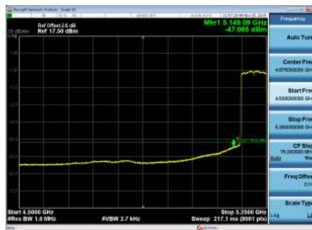
5210MHz AV
