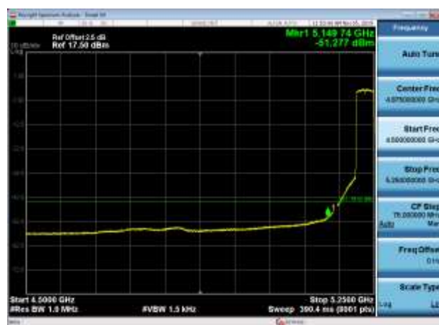
5230MHz AV
