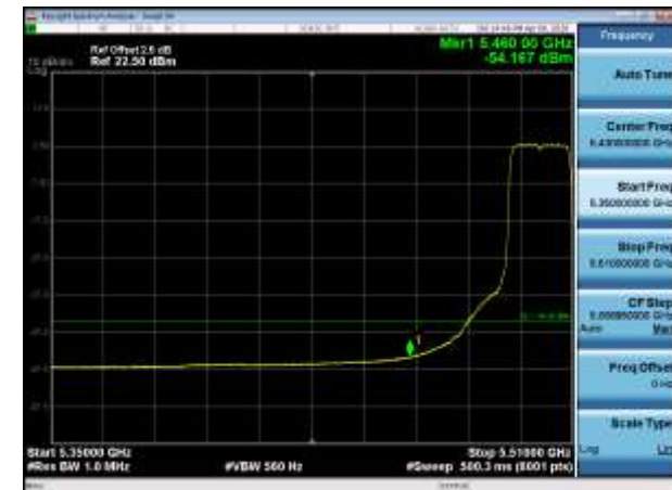
5500MHz AV
