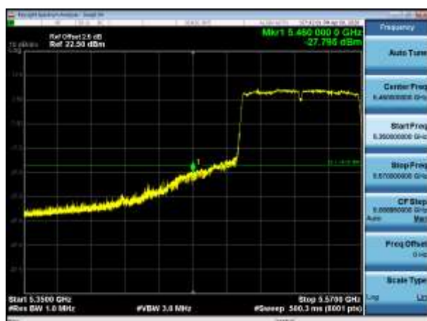
5530MHz PK
