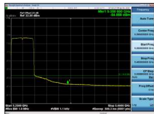
5270MHz AV
