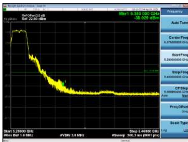
5300MHz PK
