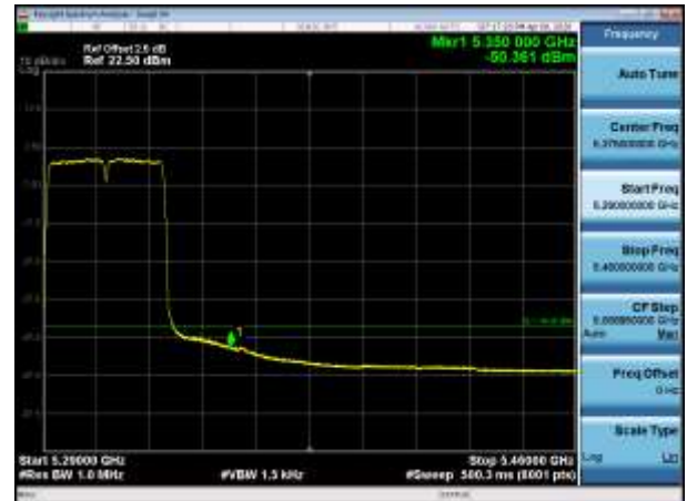
5310MHz AV
