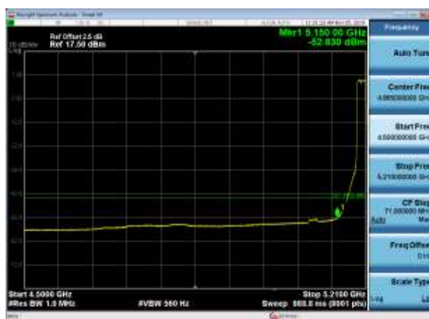
5200MHz AV
