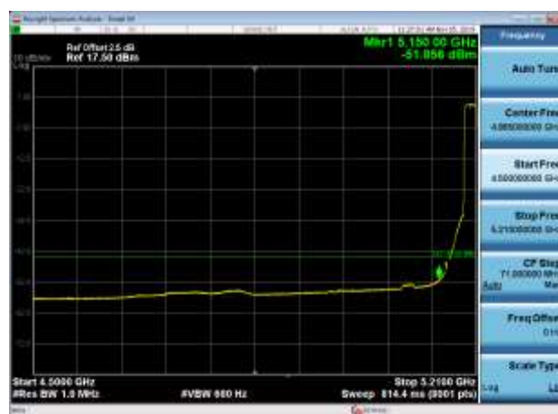
5200MHz AV
