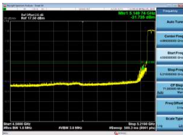
5190MHz PK
