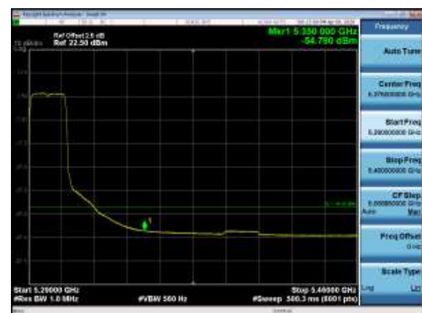
5300MHz AV
