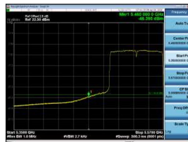
5530MHz AV
