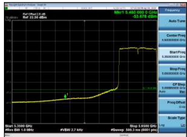
5610MHz AV
