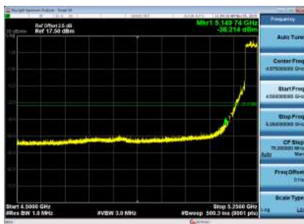
5230MHz PK
