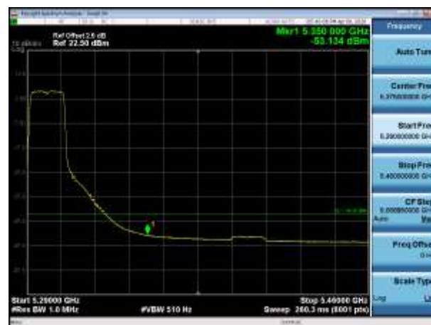
5300MHz AV
