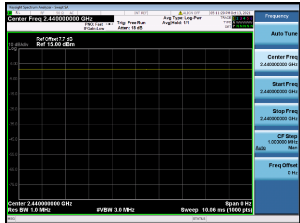
GFSK(BLE 2 Mbps)
