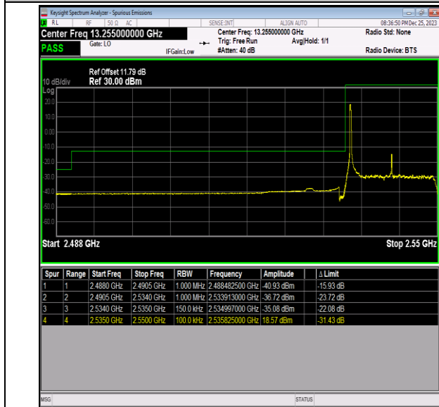
Band41_15MHz_QPSK_40115_1RB#0
