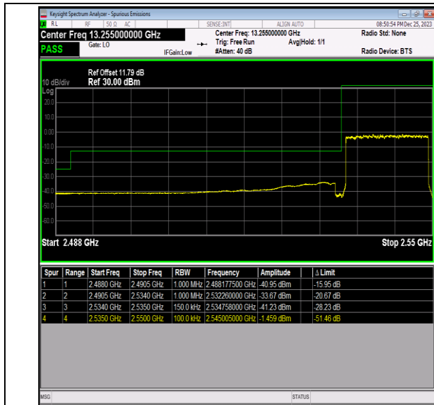
Band41_15MHz_QPSK_40115_75RB#0
