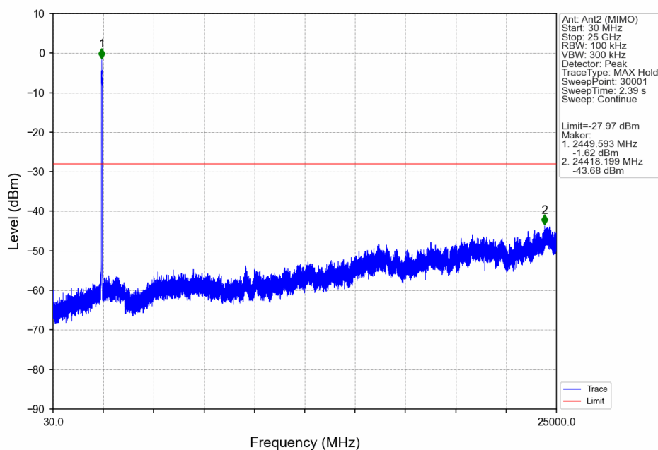
802.11ax(HEW40)_HCH_2452MHz_RU484_Left_Ant2 (MIMO)_NTNV
