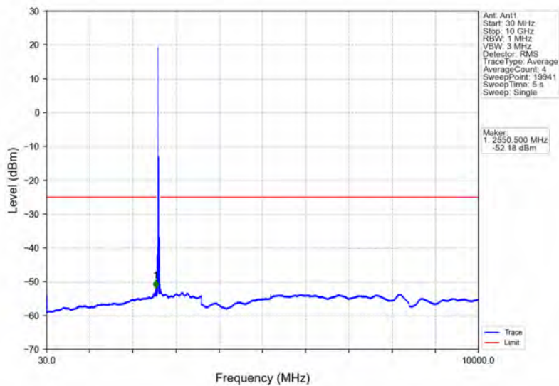
Band38_20MHz_16QAM_HCH_2610MHz_RB_1_0_NTNV
