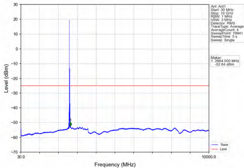
Band38_20MHz_QPSK_HCH_2610MHz_RB_1_0_NTNV
