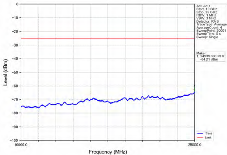
Band38_10MHz_QPSK_LCH_2575MHz_RB_1_0_NTNV
