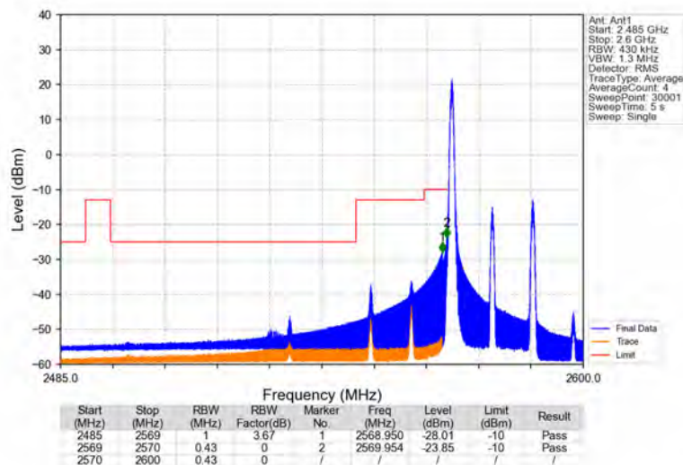
Band38_20MHz_16QAM_LCH_2580MHz_RB_1_0_NTNV
