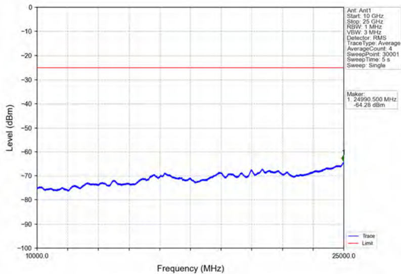
Band38_20MHz_16QAM_HCH_2610MHz_RB_1_0_NTNV
