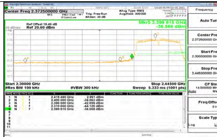
11N40MIMO_Ant1_Low_2422
