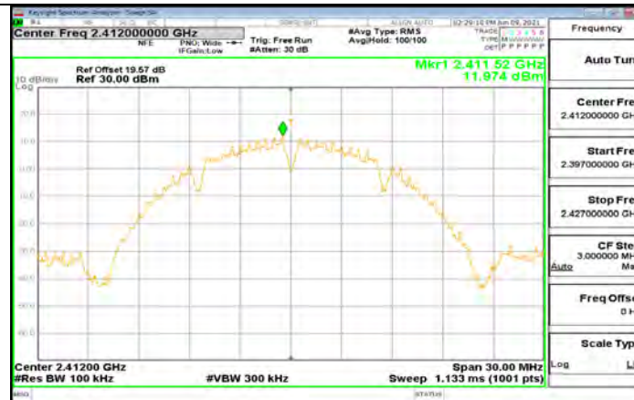
11B_Ant2_2412_0-Reference
