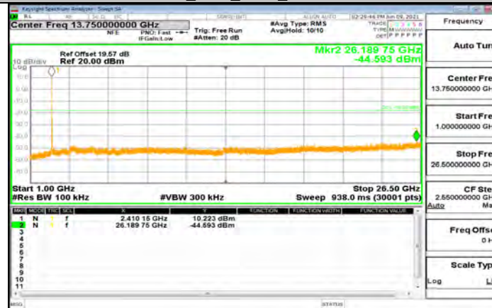
11B_Ant2_2412_1000~26500
