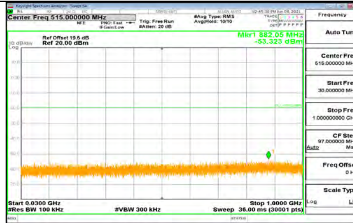
11B_Ant2_2437_30~1000
