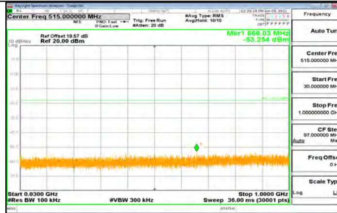
11B_Ant2_2412_30~1000
