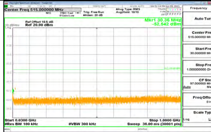
11N40MIMO_Ant2_2437_30~1000
