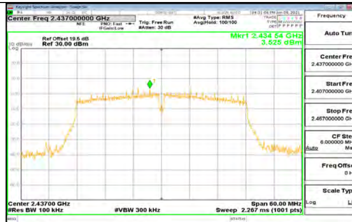
11N40MIMO_Ant2_2437_0~Reference
