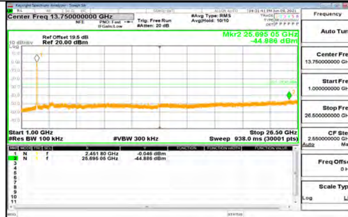
11N40MIMO_Ant2_2437_1000~26500
