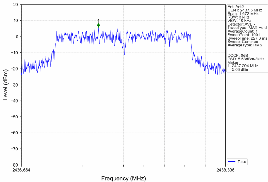
1.4M_MCH_2437.5MHz_Ant2_NTNV
