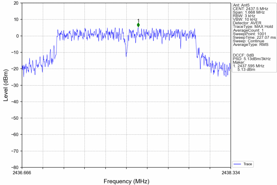
1.4M_MCH_2437.5MHz_MIMO_NTNV
