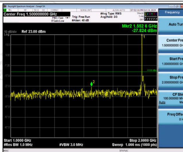
Band25-20MHz-QPSK-26590-1RB#0-Range2:1000~2000MHz
