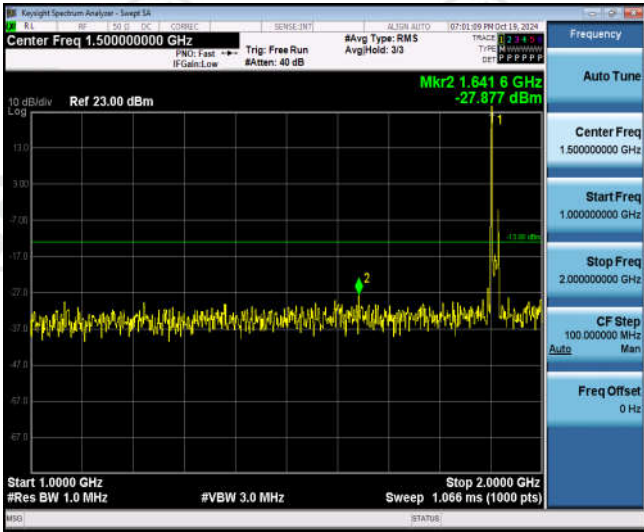
Band25-15MHz-QPSK-26615-1RB#0-Range2:1000~2000MHz
