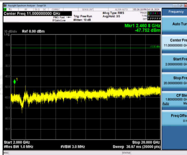
Band25-20MHz-QPSK-26365-1RB#0-Range3:2000~20000MHz
