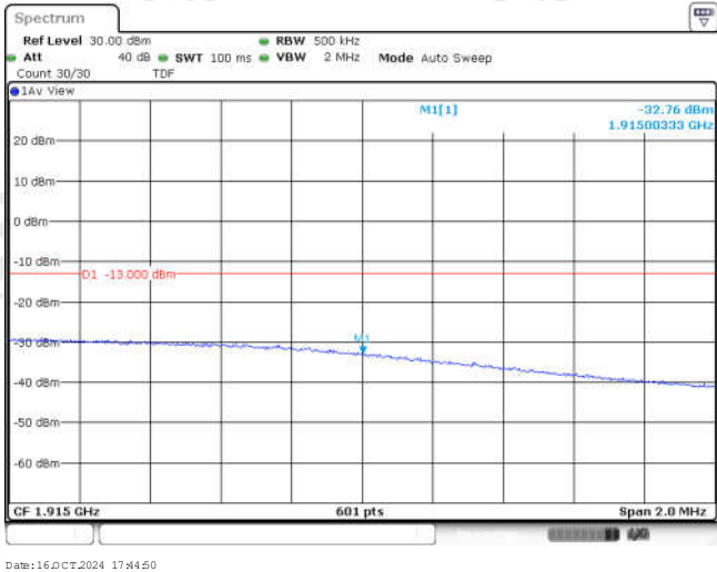
Band25-20MHz-16QAM-26590-1RB#24
