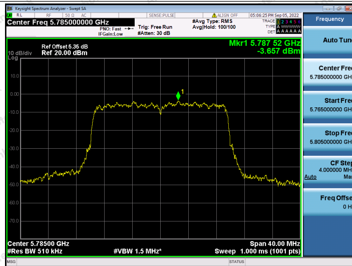
11AX20SISO_Ant2_5785
