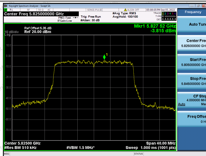
11AX20SISO_Ant2_5825
