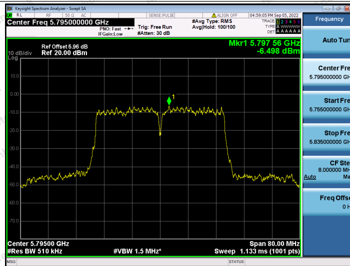
11AC40SISO_Ant2_5795
