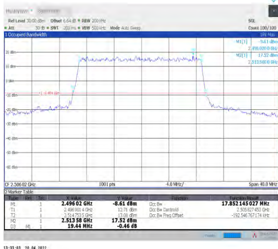
1-N41--30-20-L-1-DFT-QPSK-Outet_Full-50@0-Ant1 -17.852-19.440-≤20-PASS
