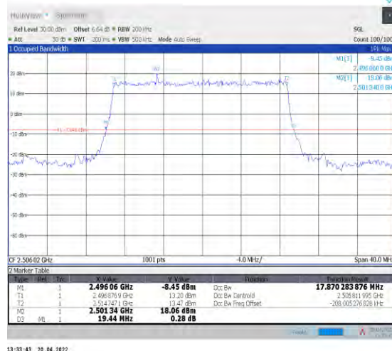
1-N41--30-20-L-2-DFT-PI2BPSK-Outet_Full-50@0-Ant1 -17.87-19.440-≤20-PASS
