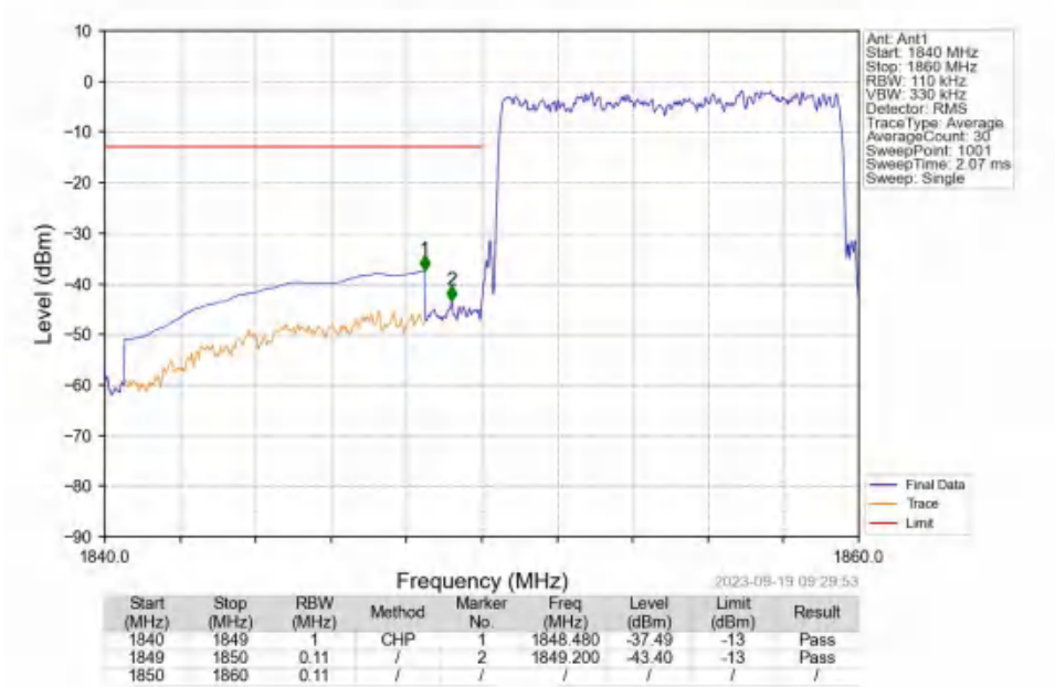
Band2_10MHz_QPSK_LCH_1855MHz_RB_50_0_NTNV
