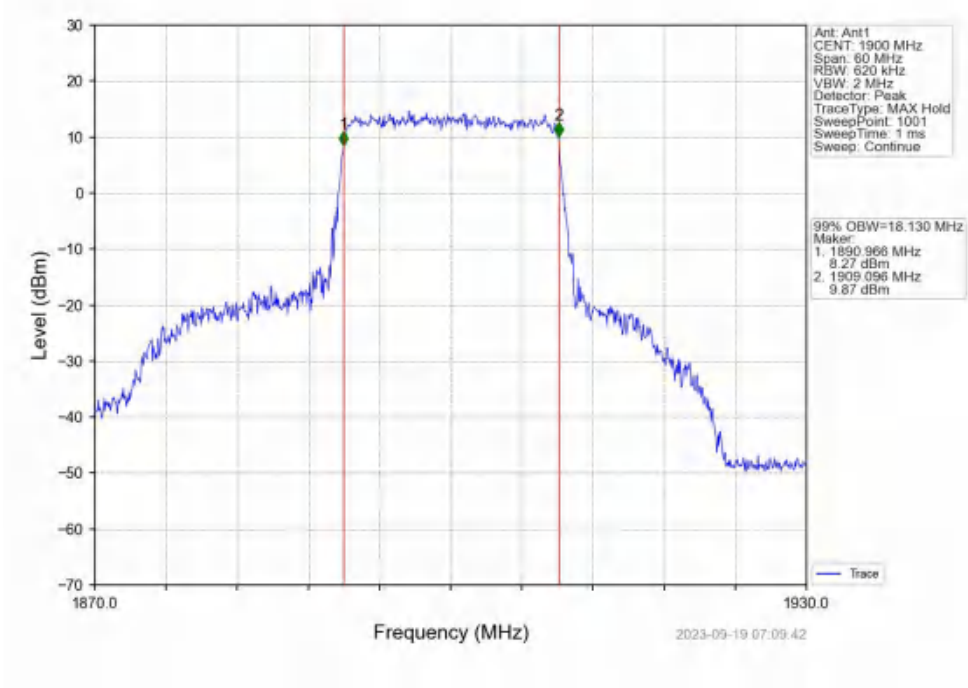
Band2_20MHz_16QAM_HCH_1900MHz_RB_100_0_NTNV
