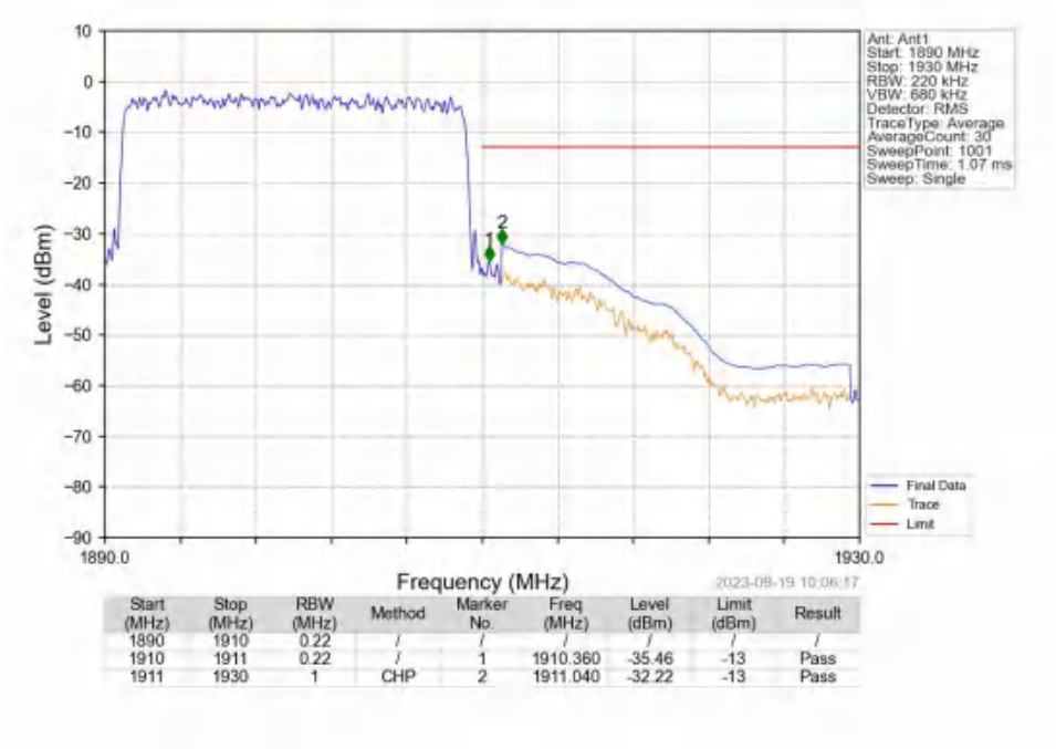
Band2_20MHz_16QAM_HCH_1900MHz_RB_100_0_NTNV
