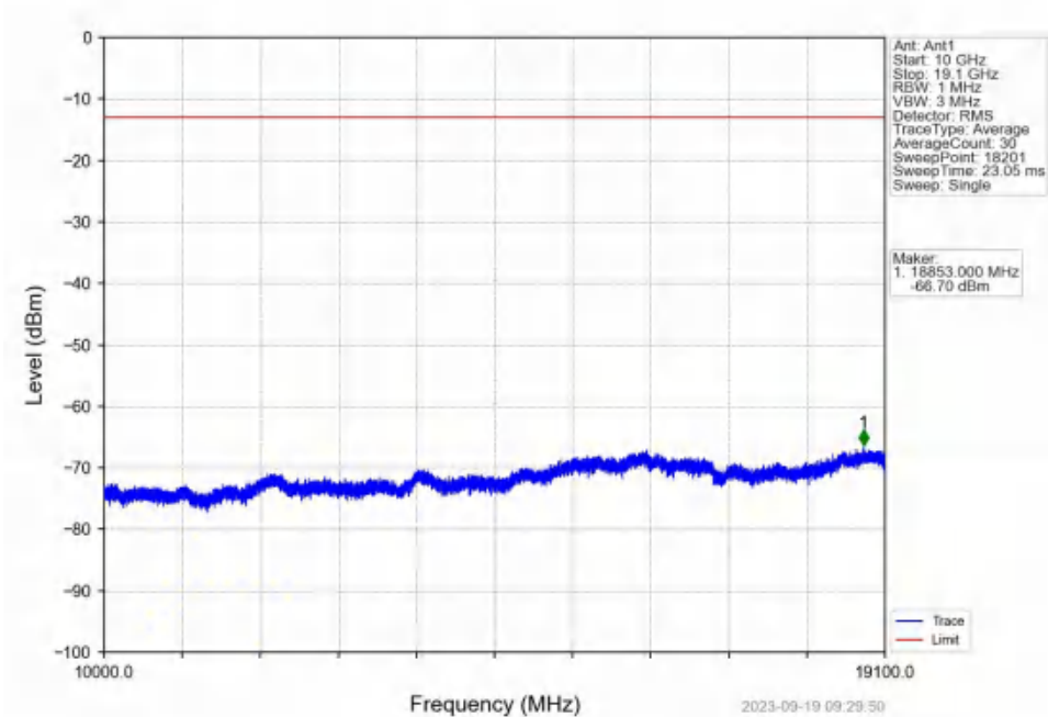
Band2_10MHz_QPSK_LCH_1855MHz_RB_1_0_NTNV
