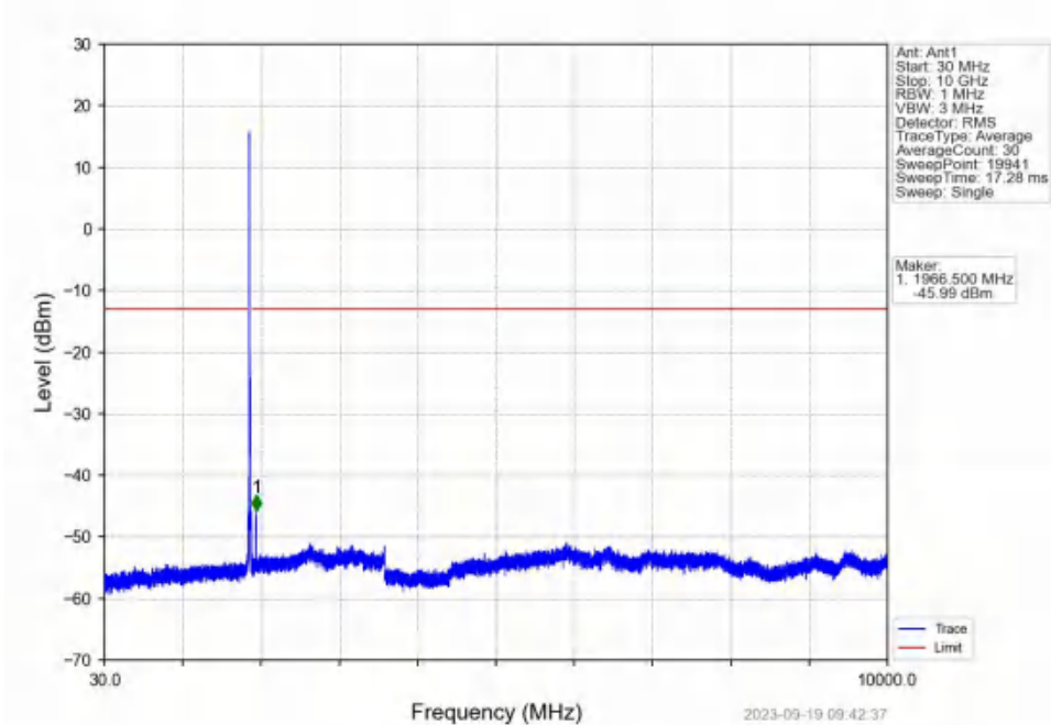
Band2_15MHz_QPSK_MCH_1880MHz_RB_1_0_NTNV
