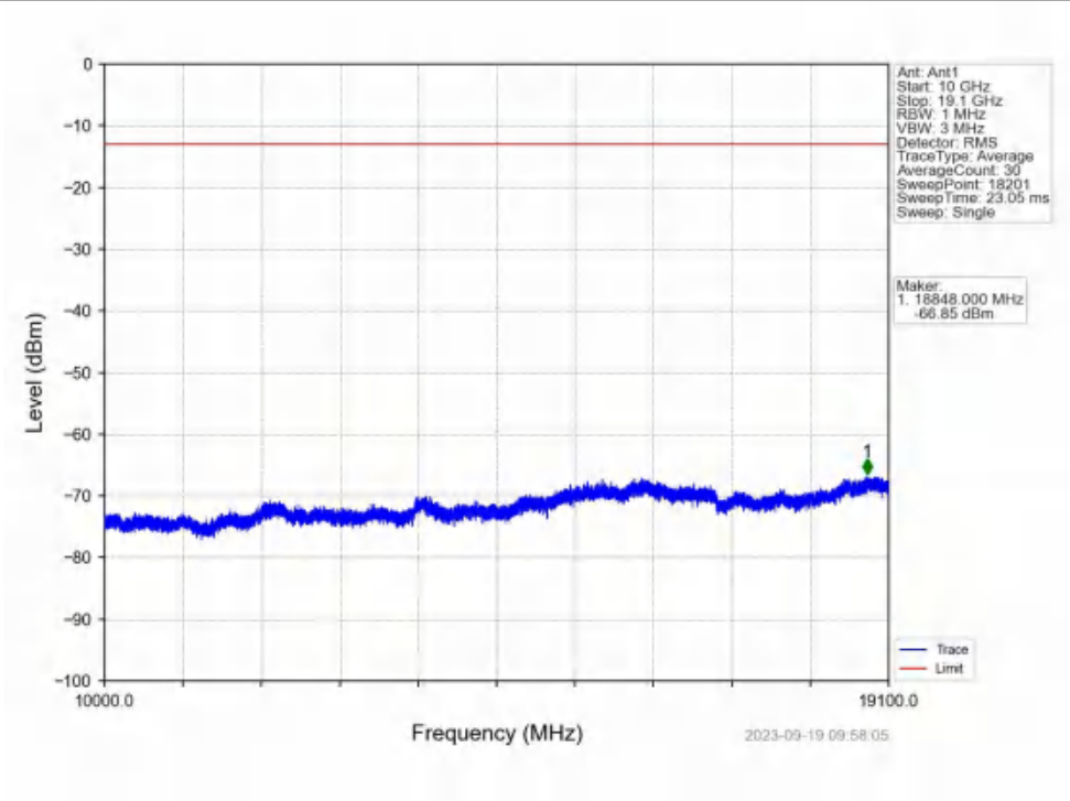
Band2_20MHz_QPSK_MCH_1880MHz_RB_1_0_NTNV
