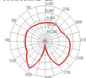
900.000MHz E2
