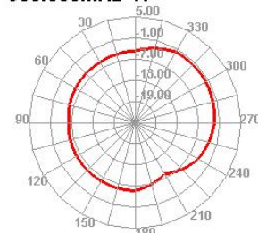
900.000MHz H
