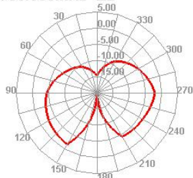
700.000MHz E2
