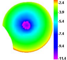
700.000MHz E1
