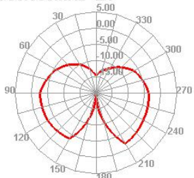
700.000MHz E1
