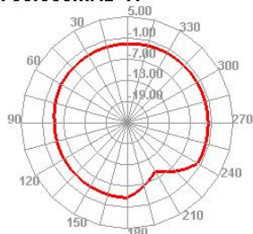
700.000MHz H
