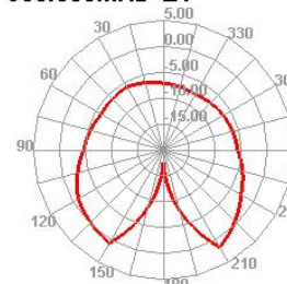
900.000MHz E1
