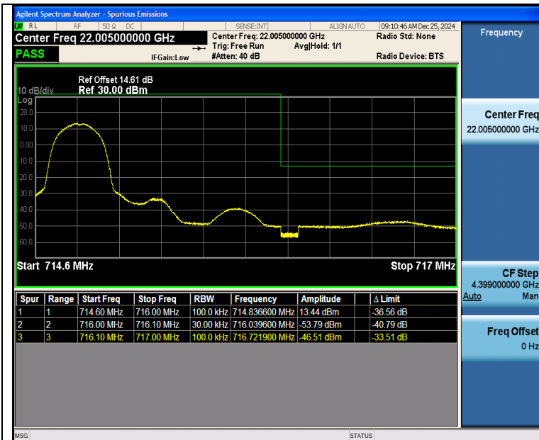
Band12 1.4MHz QPSK 23173 1RB#0
