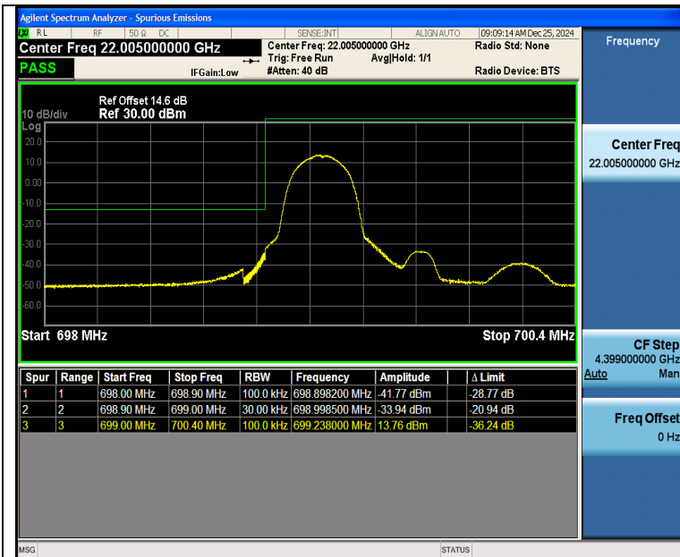
Band12 1.4MHz QPSK 23017 1RB#0
