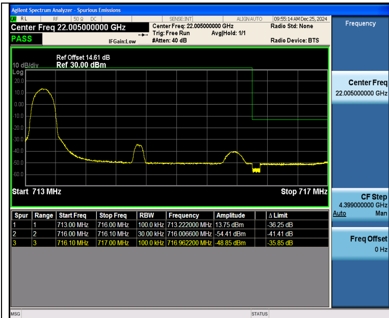
Band12 3MHz QPSK 23165 1RB#0
