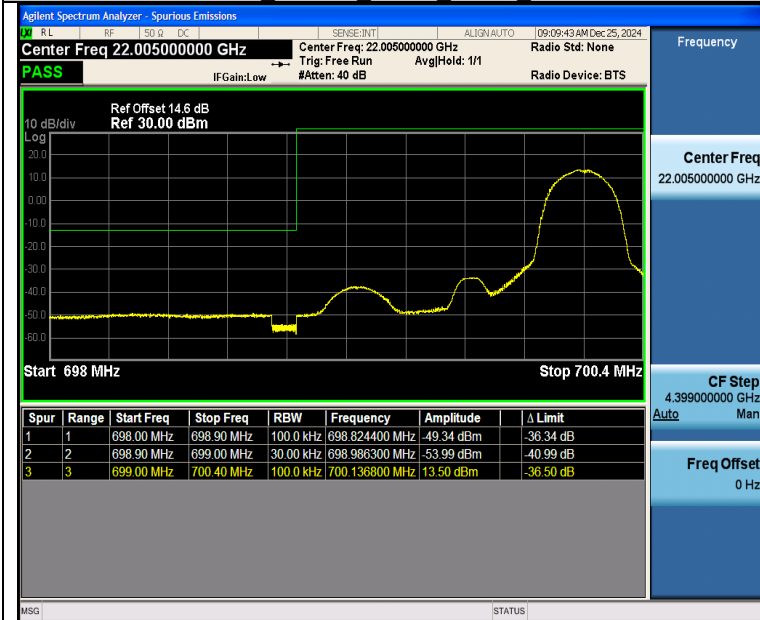
Band12 1.4MHz QPSK 23017 1RB#5
