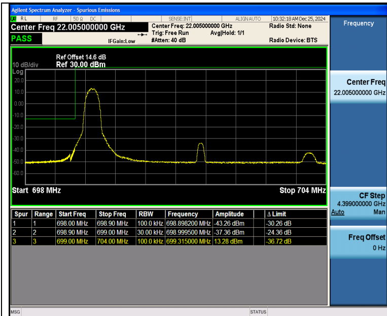
Band12 5MHz QPSK 23035 1RB#0
