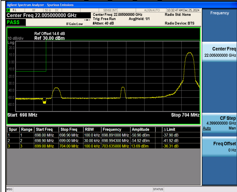
Band12 5MHz QPSK 23035 1RB#24
