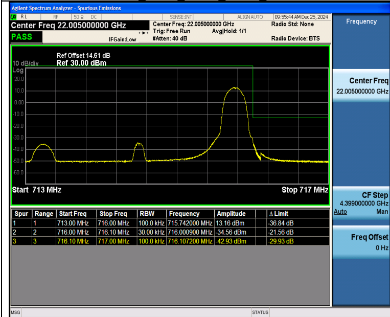
Band12 3MHz QPSK 23165 1RB#14
