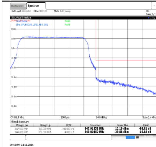
Band26(824-849)-3MHz-QPSK-26805-1RB#0-PASS
