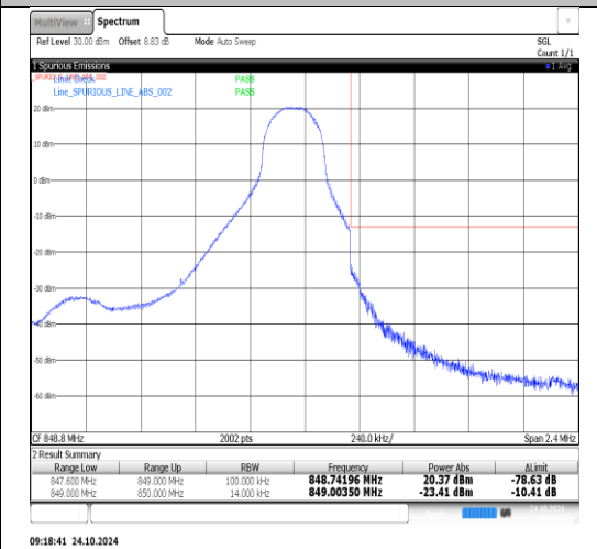
Band26(824-849)-3MHz-QPSK-26805-15RB#0-PASS
