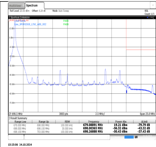
Band71-20MHz-QPSK-133372-1RB#99-PASS
