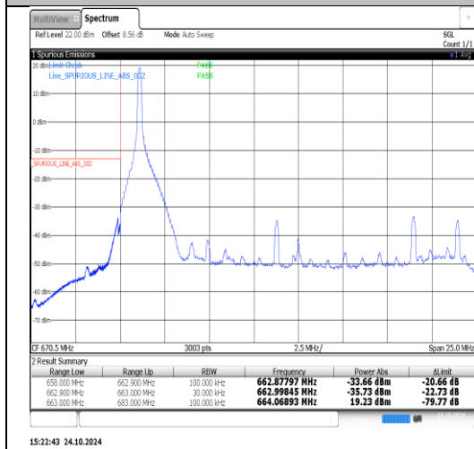
Band71-20MHz-QPSK-133222-1RB#99-PASS
