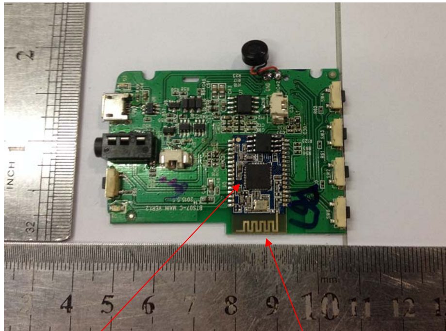
Bluetooth module
