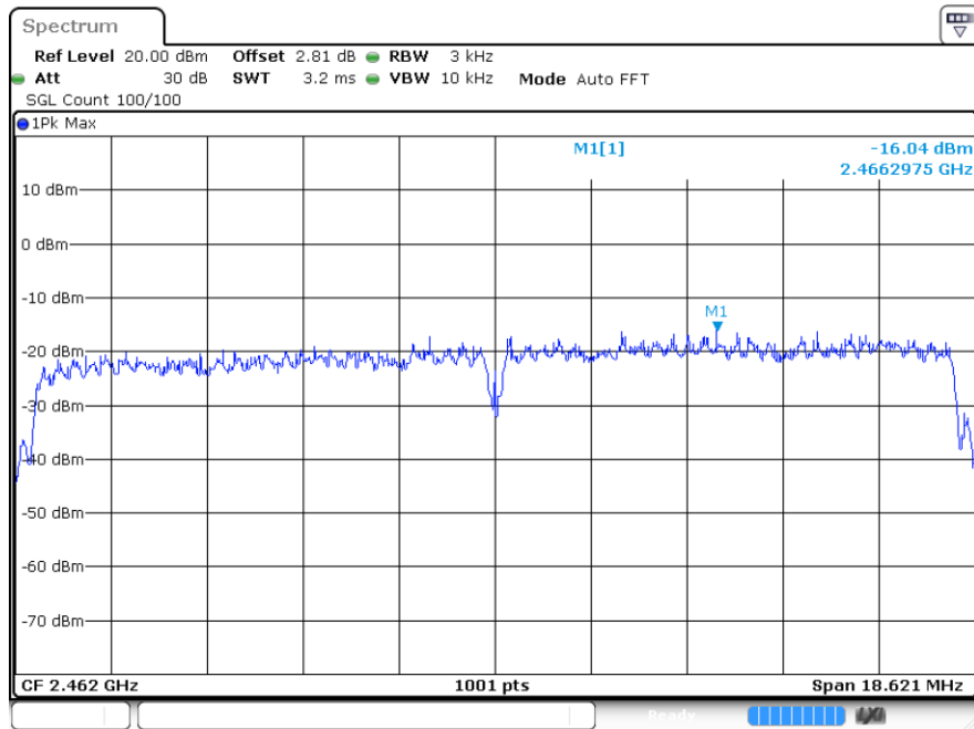
Test_Graph_802.11n20_ANT1_2462
