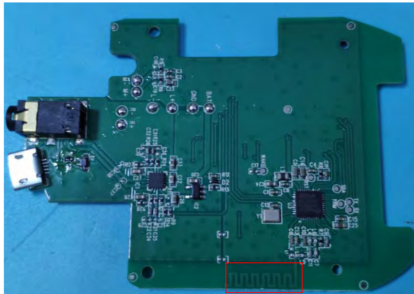
Antenna
