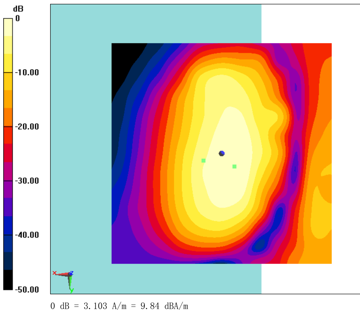
Fig B.8 T-Coil WCDMA 1900
