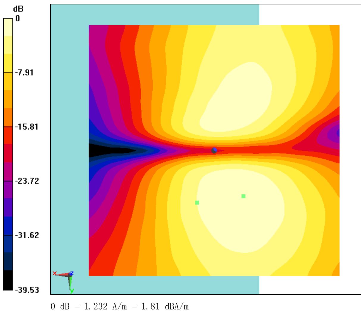
Fig B.7 T-Coil WCDMA 1900
