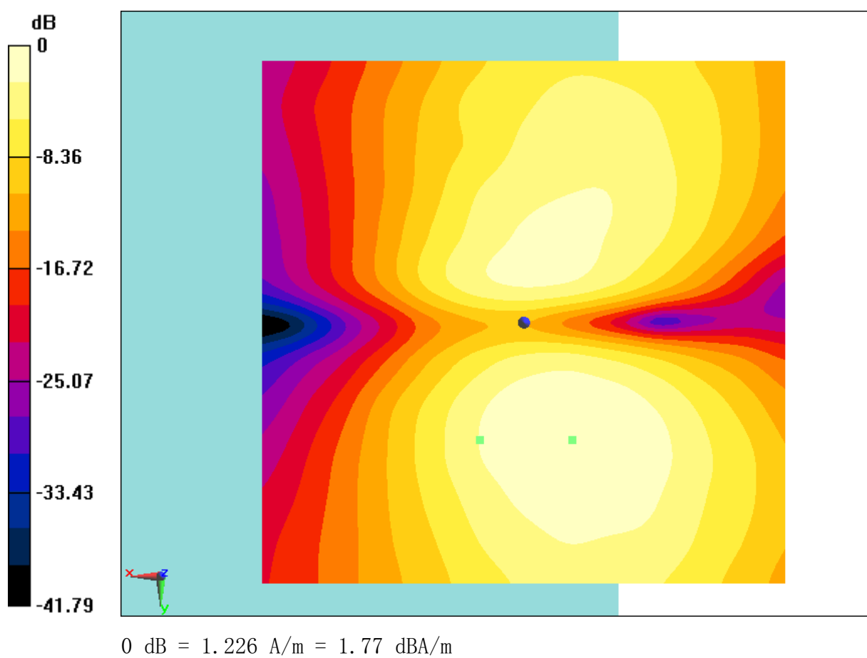
Fig B.9 T-Coil WCDMA 1700
