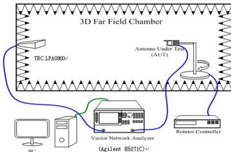
图 1. 微波暗室内仪器设置 r.
