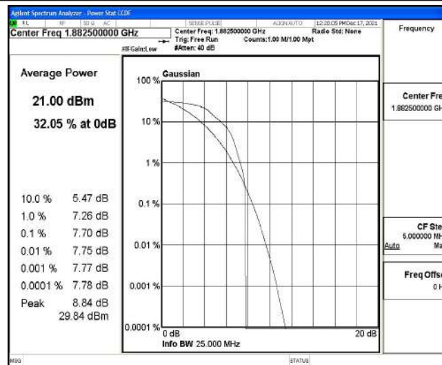
Band25-10MHz-QPSK-26365-1-0-Low-7.70-7.70-13-PASS
