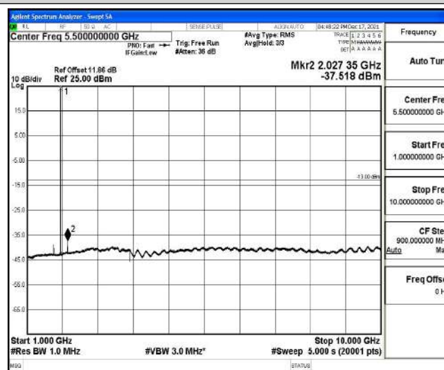
Band25-10MHz-QPSK-26090-1-0-Low-1000-10000--37.52-PASS
