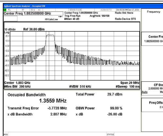
Band25-10MHz-QPSK-26365-6-0-Low-1.3559-2.807-PASS
