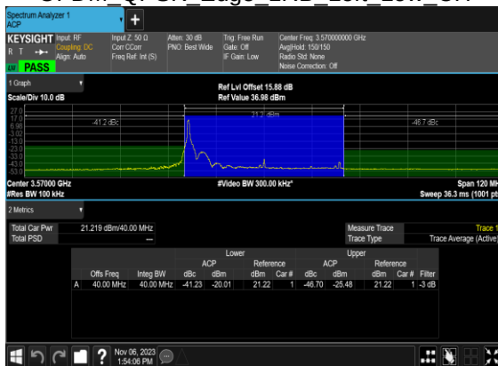
N48(40M)_DFT-s-OFDM QPSK Edge 1RB Left Low CH
