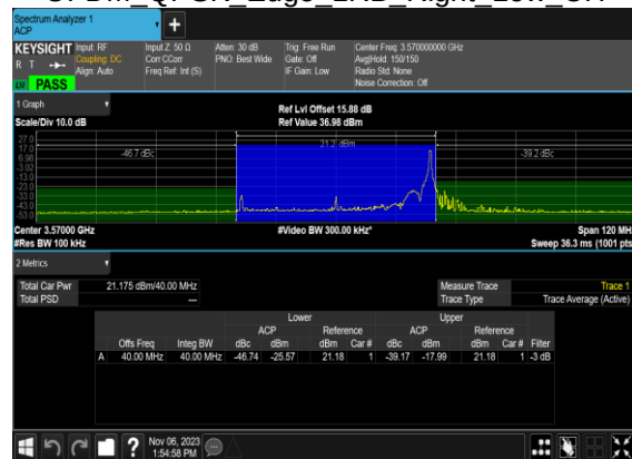
N48(40M)_DFT-s-OFDM QPSK Edge 1RB Right Low CH
