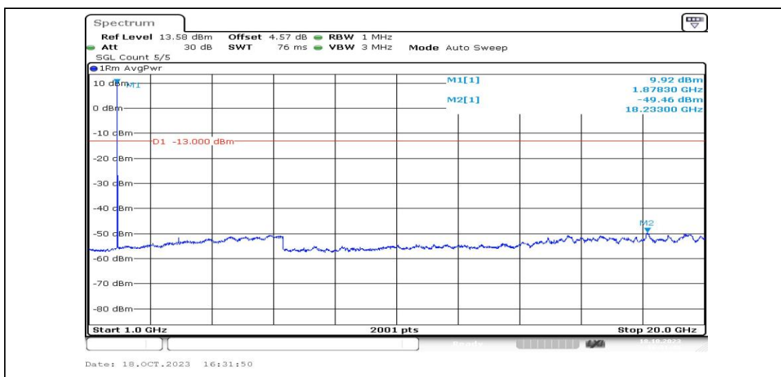
Band25-3MHz-QPSK-26365-1RB#0-Range4:1000~20000MHz-PASS
