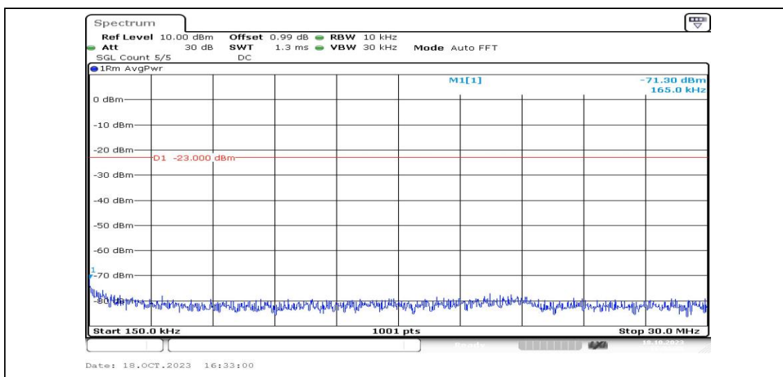
Band25-3MHz-QPSK-26675-1RB#0-Range2:0.15~30MHz-PASS
