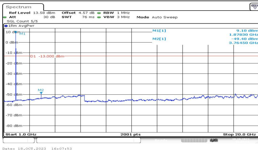
Band25-1.4MHz-QPSK-26365-1RB#0-Range4:1000~20000MHz-PASS
