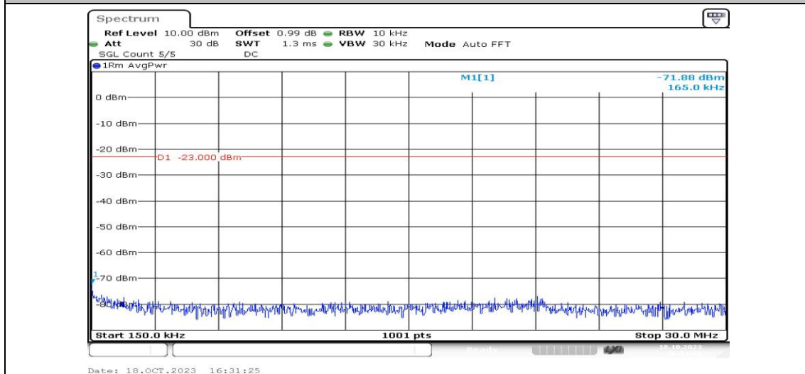
Band25-3MHz-QPSK-26365-1RB#0-Range2:0.15~30MHz-PASS
