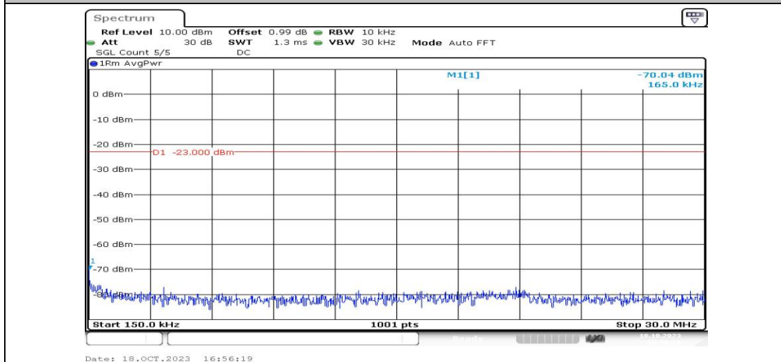
Band25-5MHz-QPSK-26365-1RB#0-Range2:0.15~30MHz-PASS
