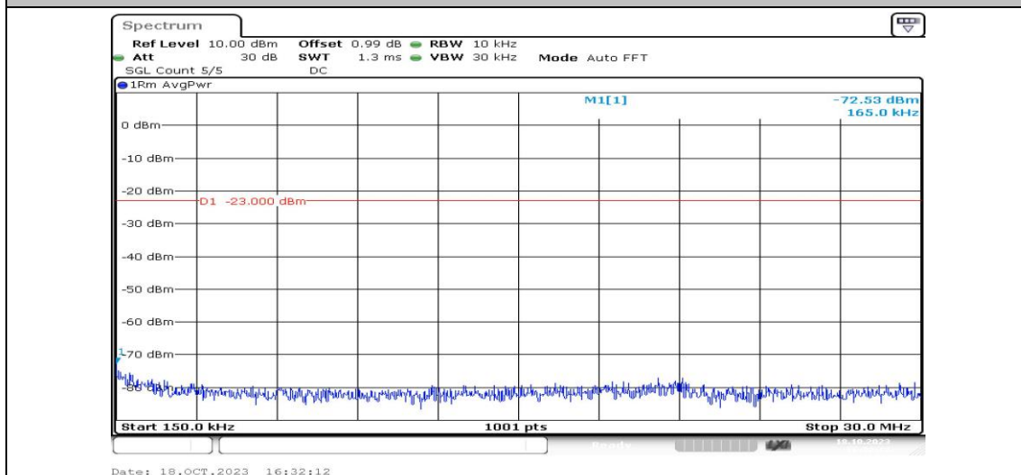
Band25-3MHz-16QAM-26365-1RB#0-Range2:0.15~30MHz-PASS
