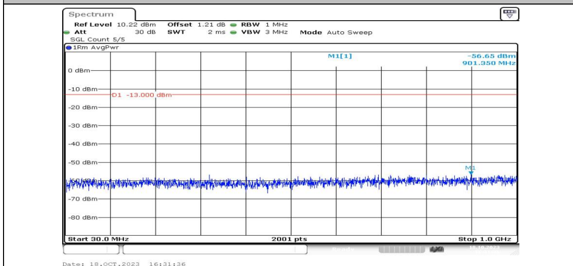
Band25-3MHz-QPSK-26365-1RB#0-Range3:30~1000MHz-PASS
