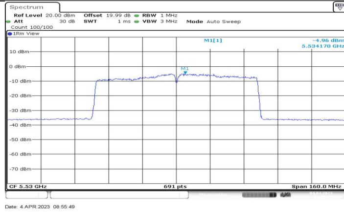
11AC80MIMO_Ant0_5530
