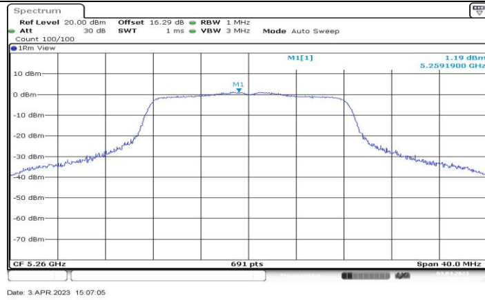
11A_Ant0_5260
