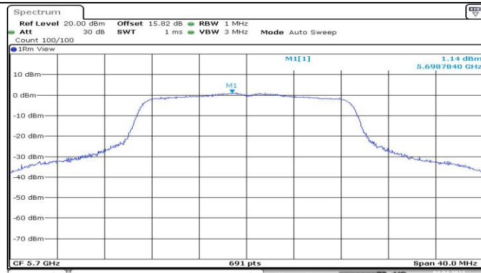
11N20MIMO_Ant1_5700
