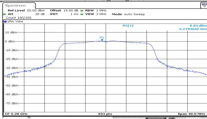
11N20MIMO_Ant0_5280
