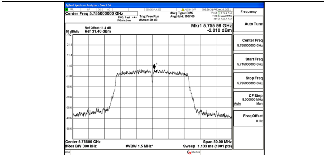
11N40MIMO_Ant2_5755
