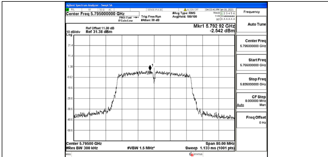
11AC40MIMO_Ant2_5795
