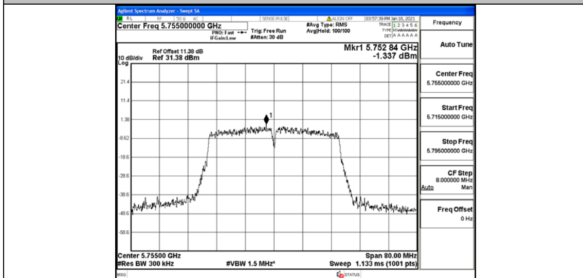
11AC40MIMO_Ant2_5755
