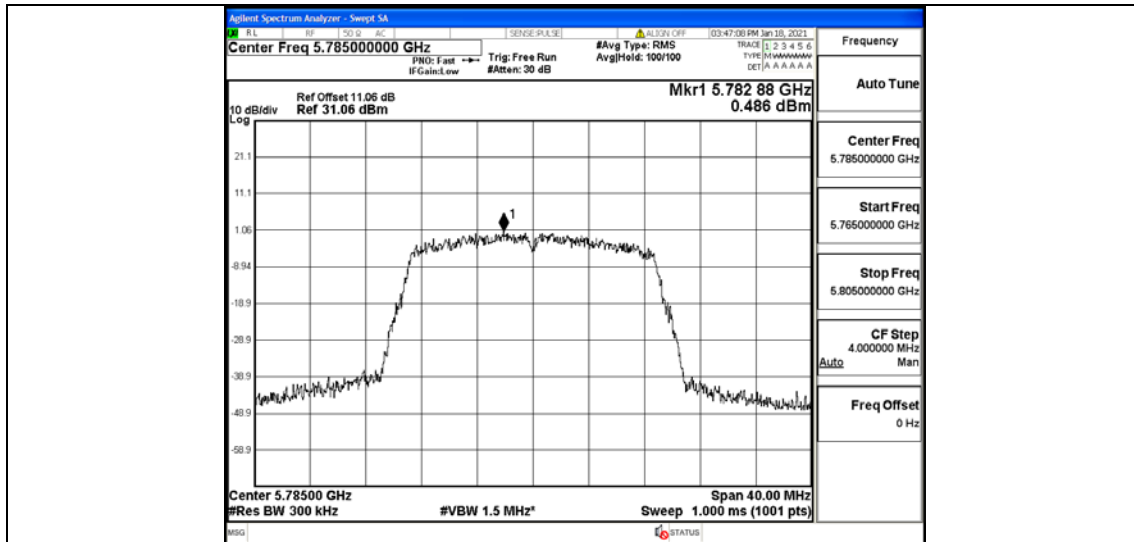
11AC20MIMO_Ant2_5785
