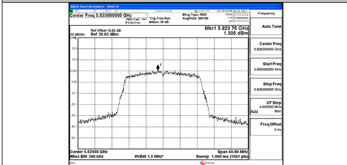
11N20MIMO_Ant2_5825
