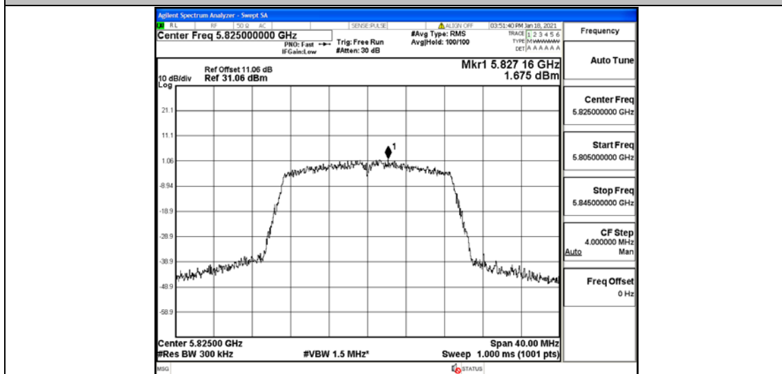
11AC20MIMO_Ant2_5825
