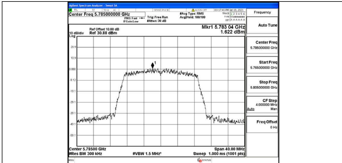
11N20MIMO_Ant1_5825
