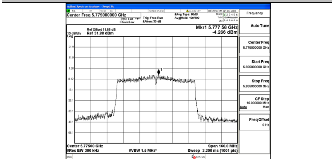
11AC80MIMO_Ant2_5775
