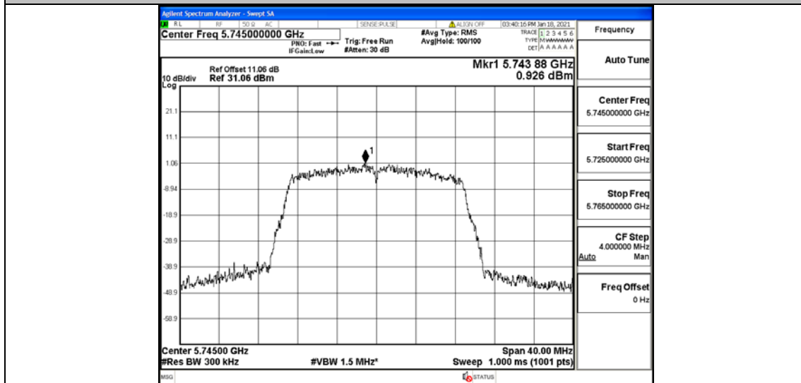
11AC20MIMO_Ant2_5745
