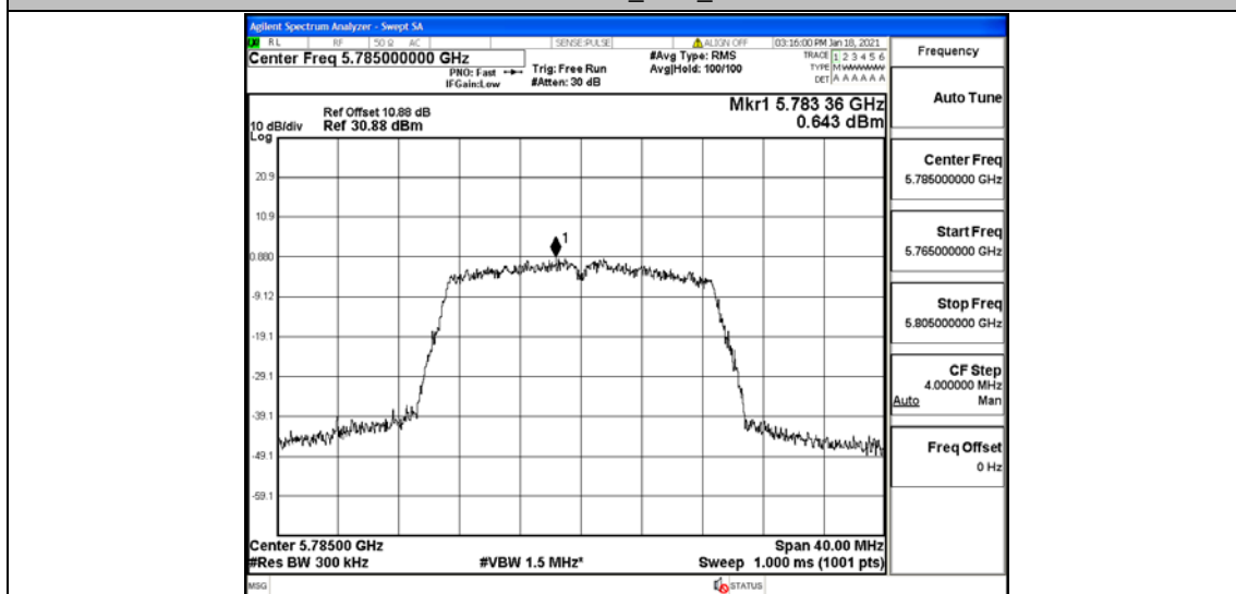
11N20MIMO_Ant2_5785
