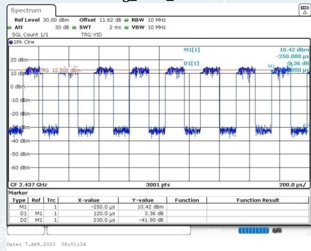
802.11g_Ant1_2437MHz
