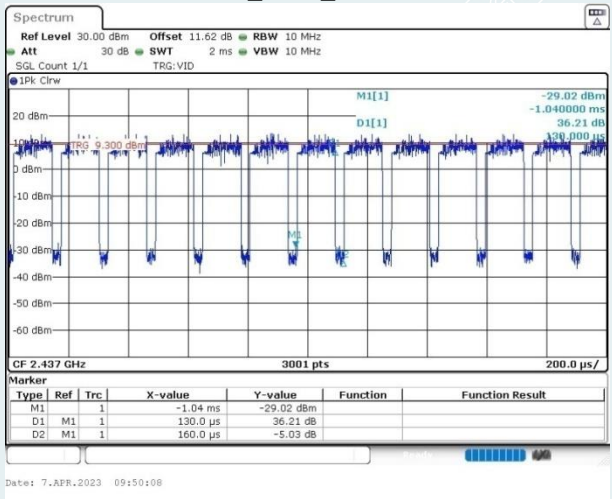
VHT40_Ant1_2437MHz
