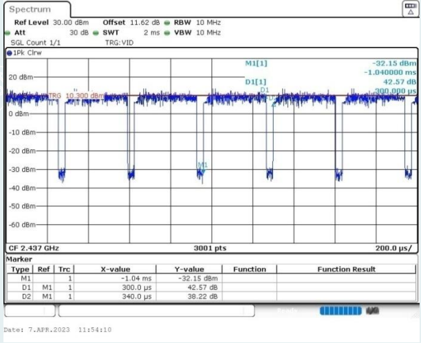
802.11ax HE40_Ant1_2437MHz
