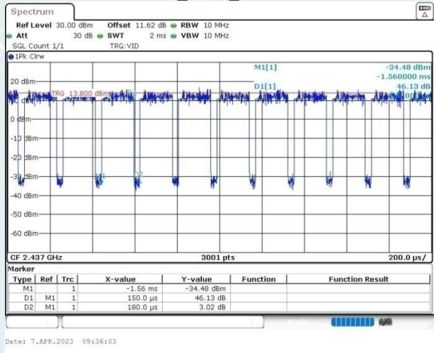
VHT20_Ant1_2437MHz
