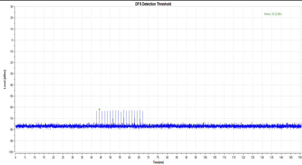
20M_5320_Type1
