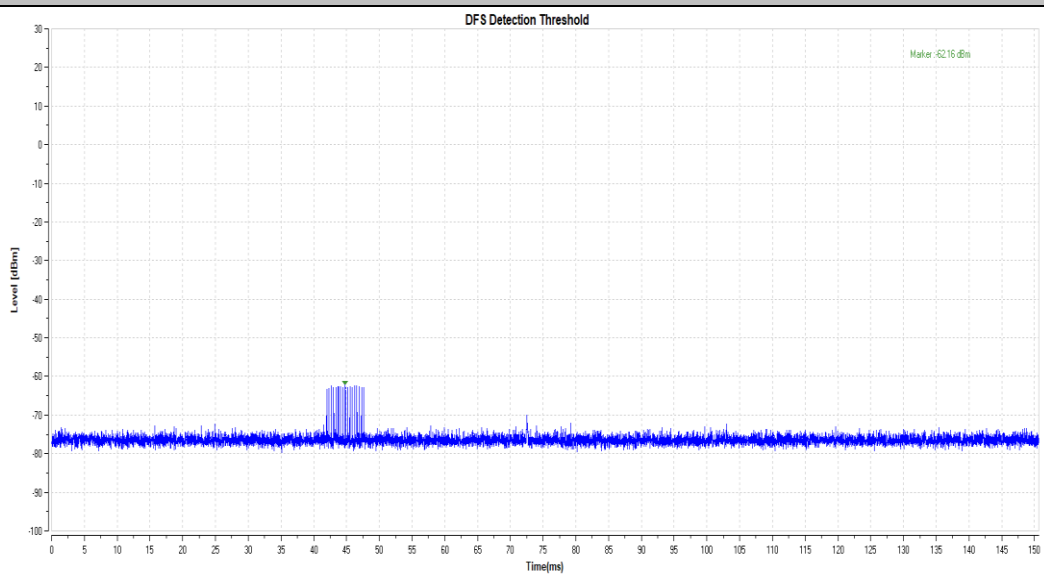
40M_5510_Type3
